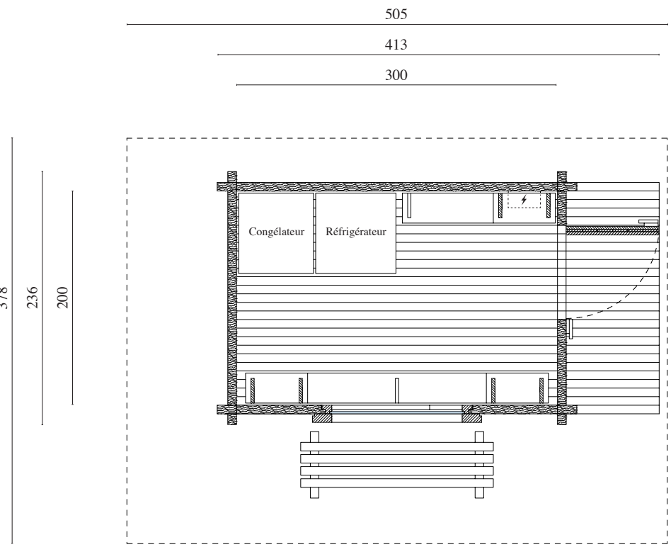
Plan 1:50
