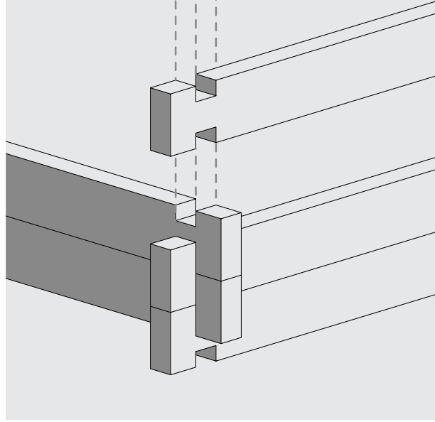
Schéma de l'assemblage à mi-bois de la construction en madrier
