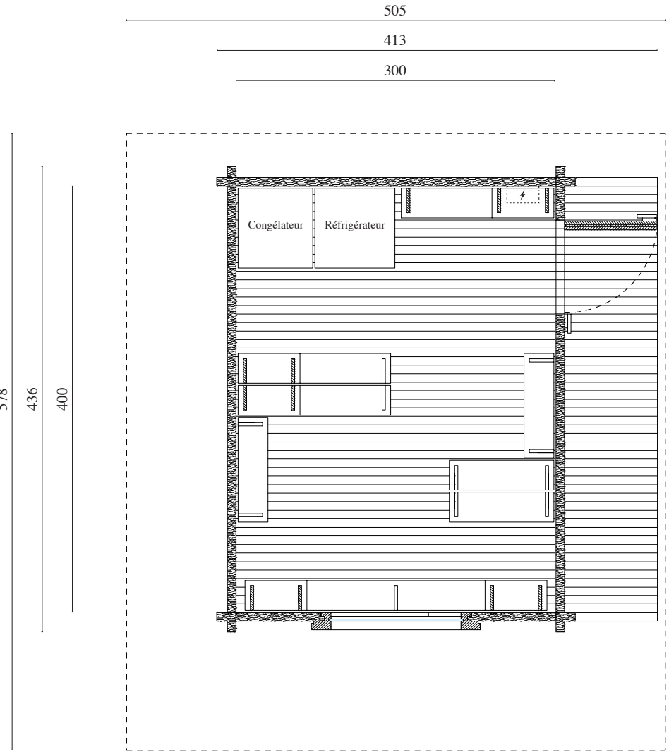
Plan 1:50
