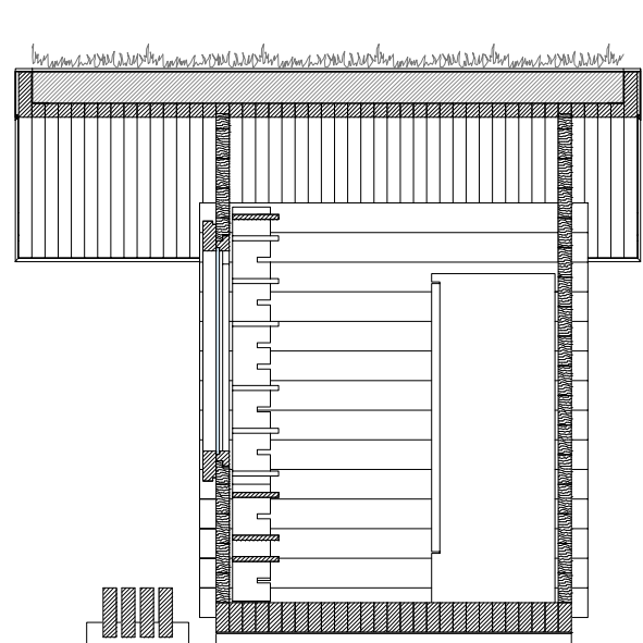
Coupe longitudinale 1:50
