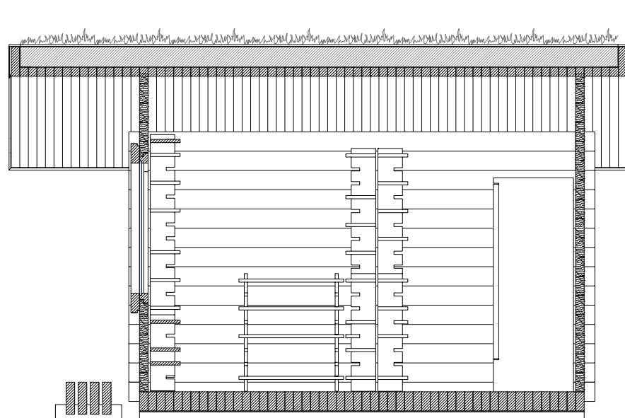
Coupe longitudinale 1:50
