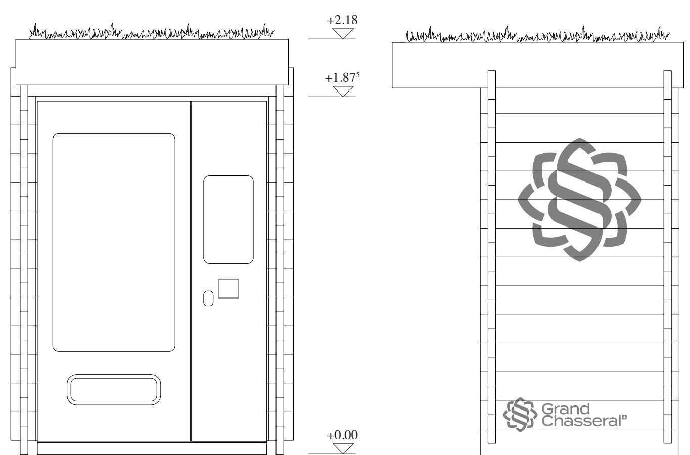
Élévation frontale 1:20
