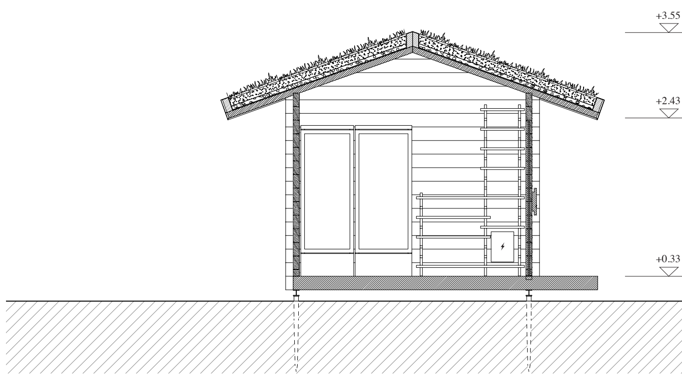
Coupe transversale 1:50
