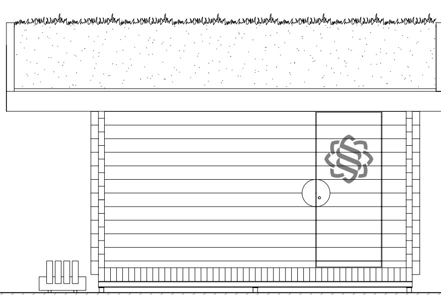
Élévation latérale 1:50
