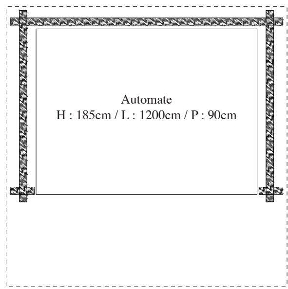
Plan 1:20
