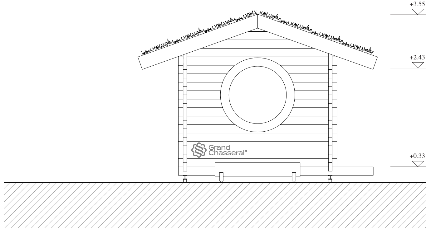
Élévation frontale 1:50
