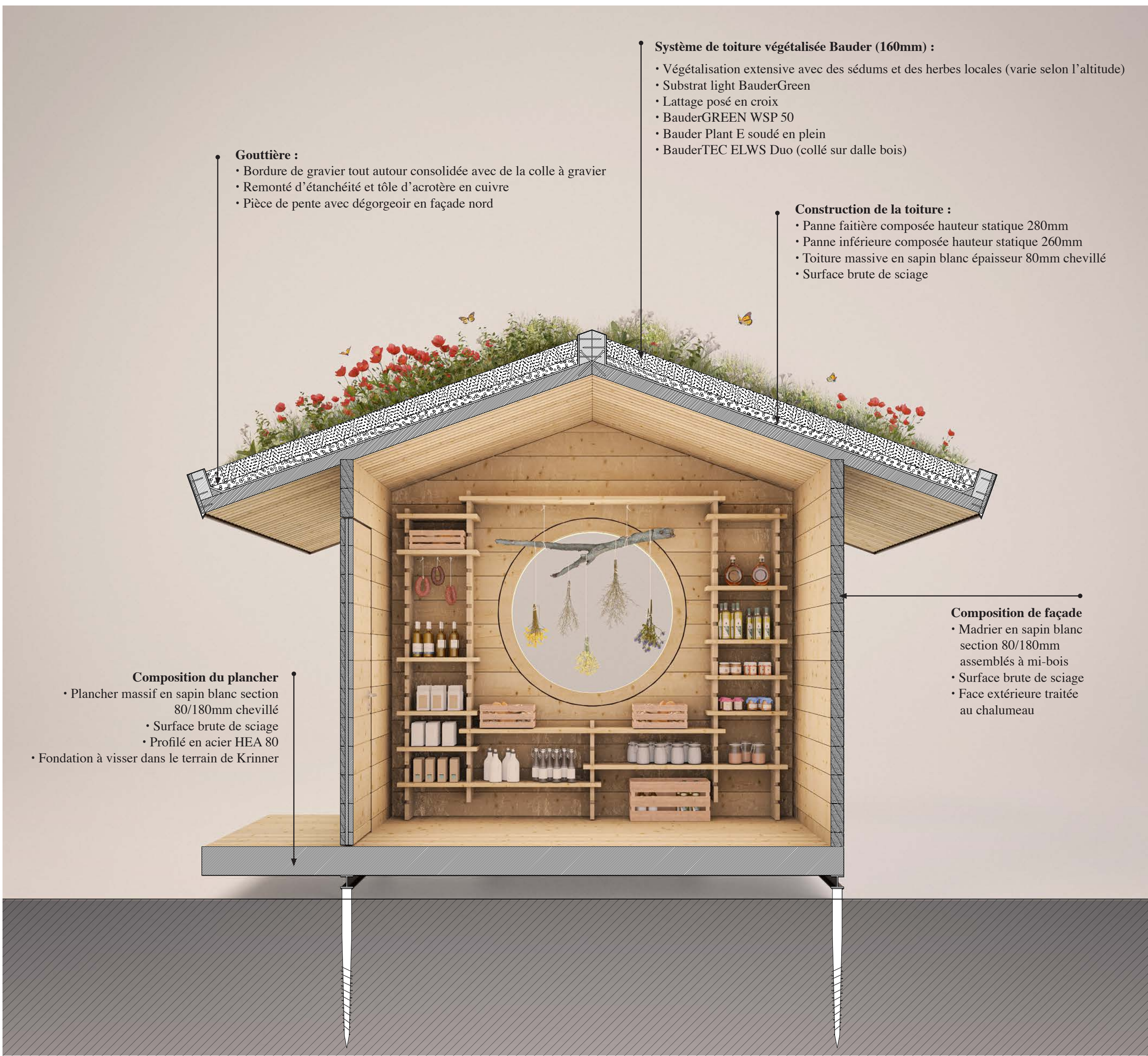
Coupe transversale 1:20
