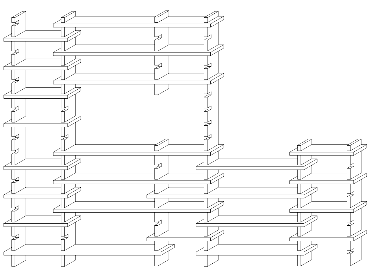
Axonométrie 1:20
