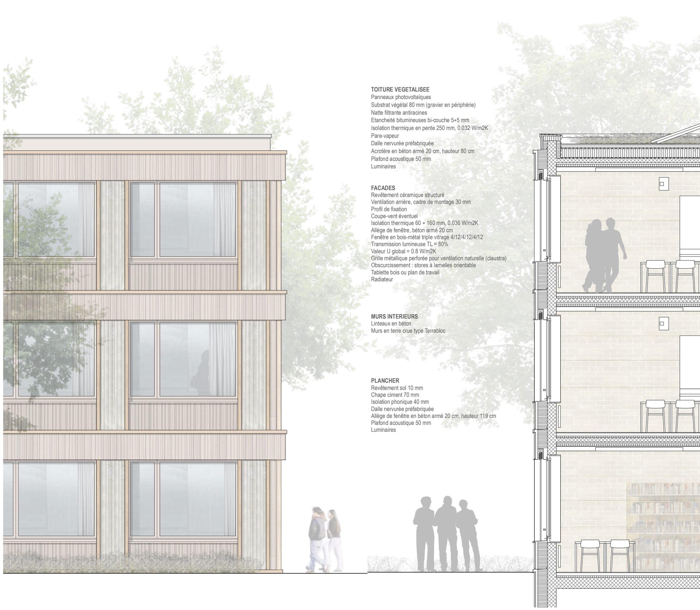
Détail constructif 1:50
