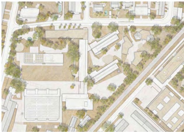
Situationsplan mit Dachschieferdach, 1:500
