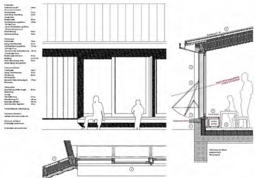
1:20 DETAILSCHNITT
