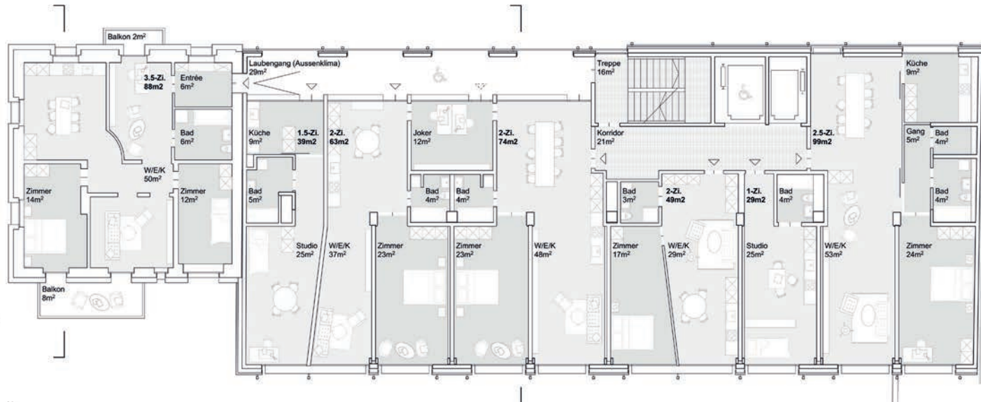
Wohnungstypen 1:200
