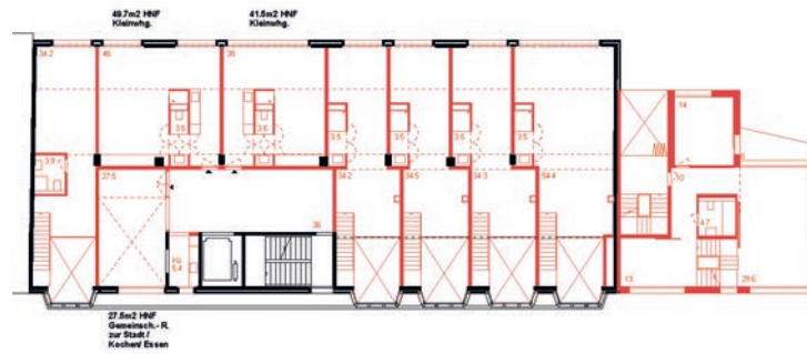
2.Obergeschoss 1:500
