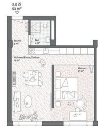
2.5 Zi-Wohnung, 53m² 2-4.OG
