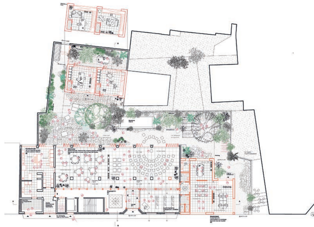
Erdgeschoss 1:500
