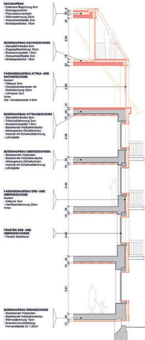
Fassadenschnitt Nordfassade De Boni
