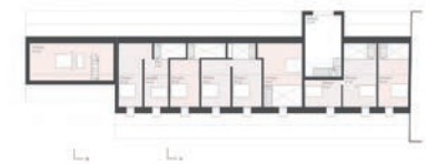
2.Dachgeschoss 1:1000
