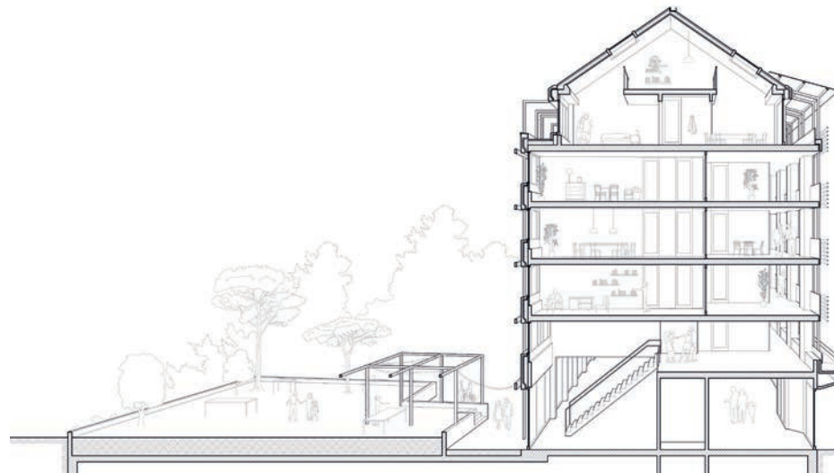
Schnittperspektive
