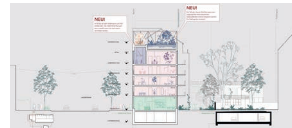
Schnitt D-D 1:1000
