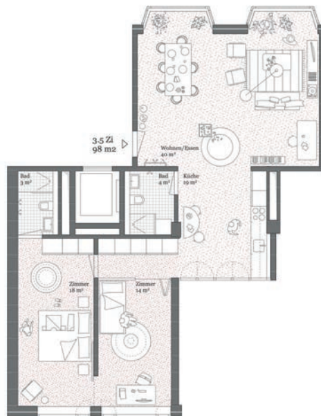
Wohungstyp 1:100 3.5 Zi-Wohnung, 98m² 2,4.OG
