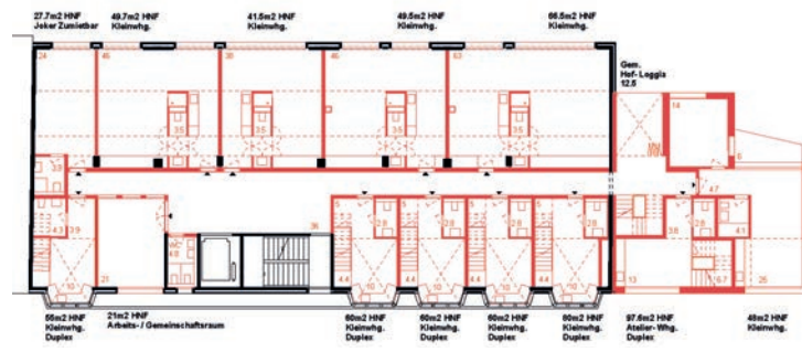
1.Obergeschoss 1:500
