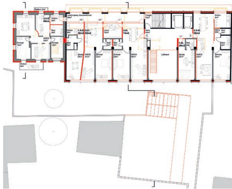
1.Obergeschoss 1:500
