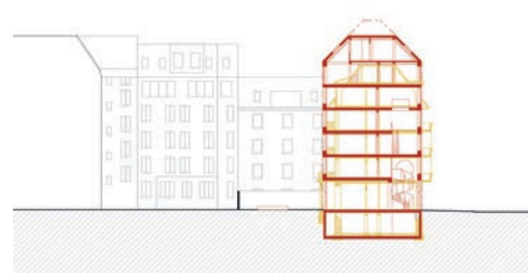
Schnitt BB 1:1000
