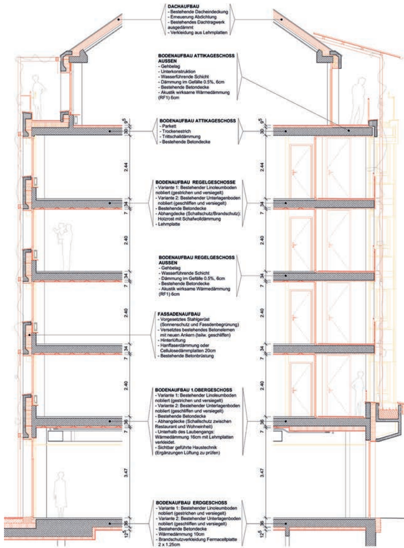
Fassadenschnitt Südfassade Erlenhof
