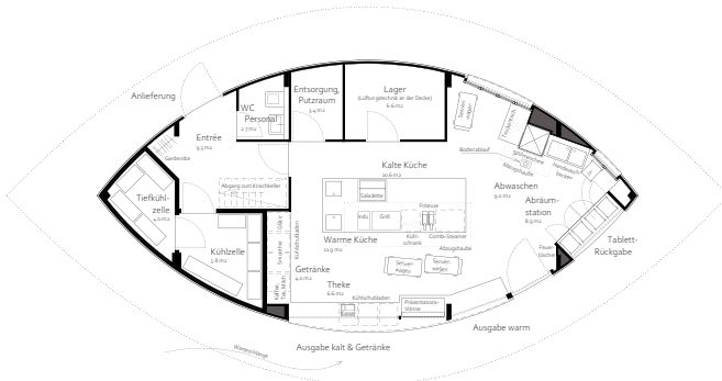
Gastrogebäude 1:250
