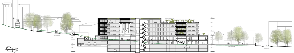
COUPE LONGITUDINALE 1:500
