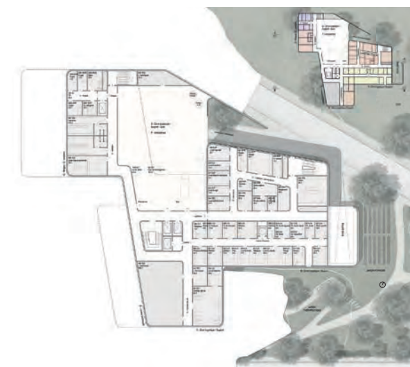
Plan -01 1 / 200
