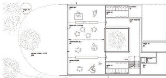
crèche - nurserie - LIAVE - rez-de-chaussée inf. 1:200
