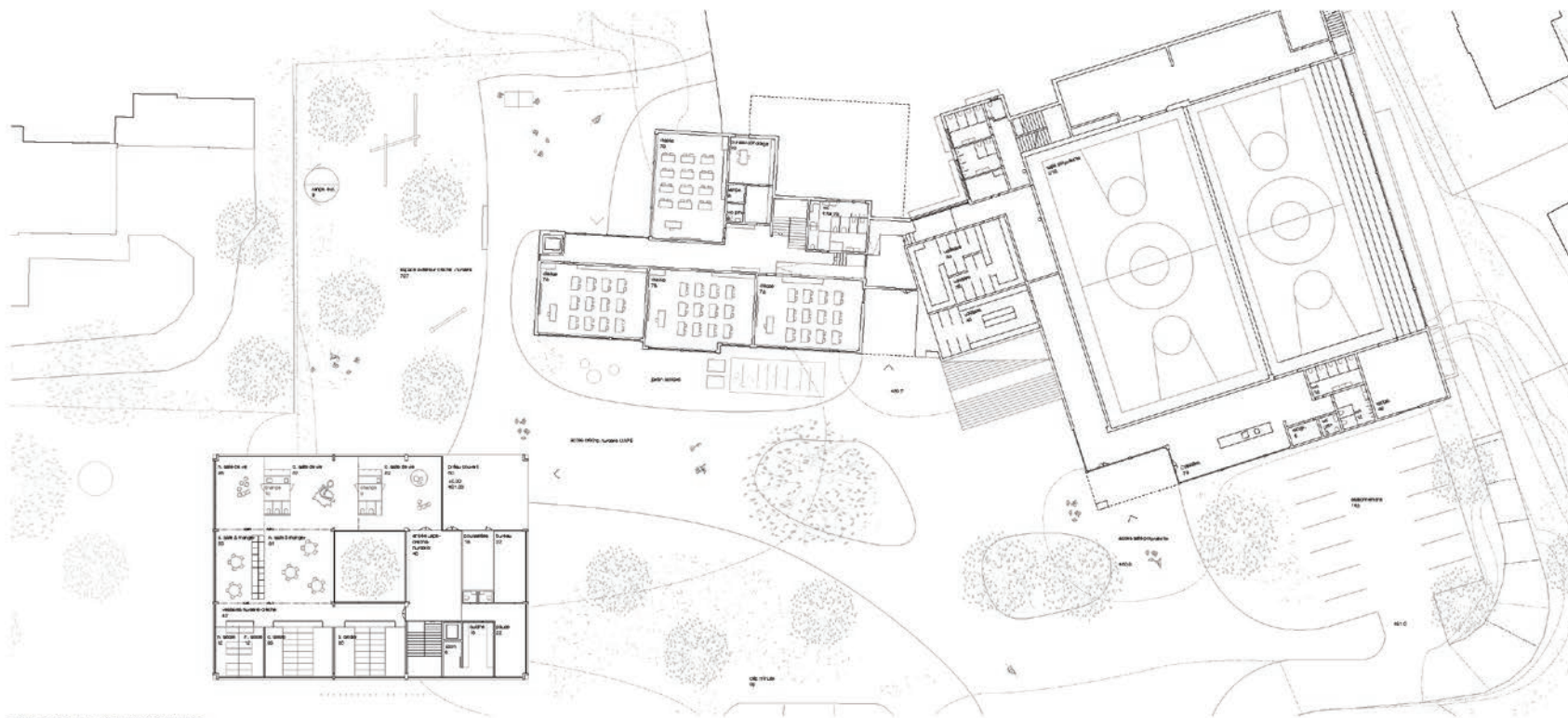
crèche - nurserie - LIAVE - rez-de-chaussée intermédiaire 1:200
