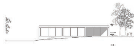
crèche - nurserie - LIAVE - façade est 1:200
