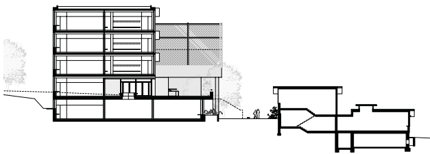
Querschnitt 1:800
