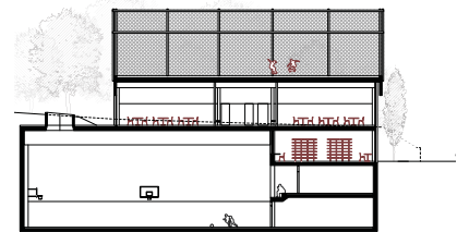
Querschnitt 1:800
