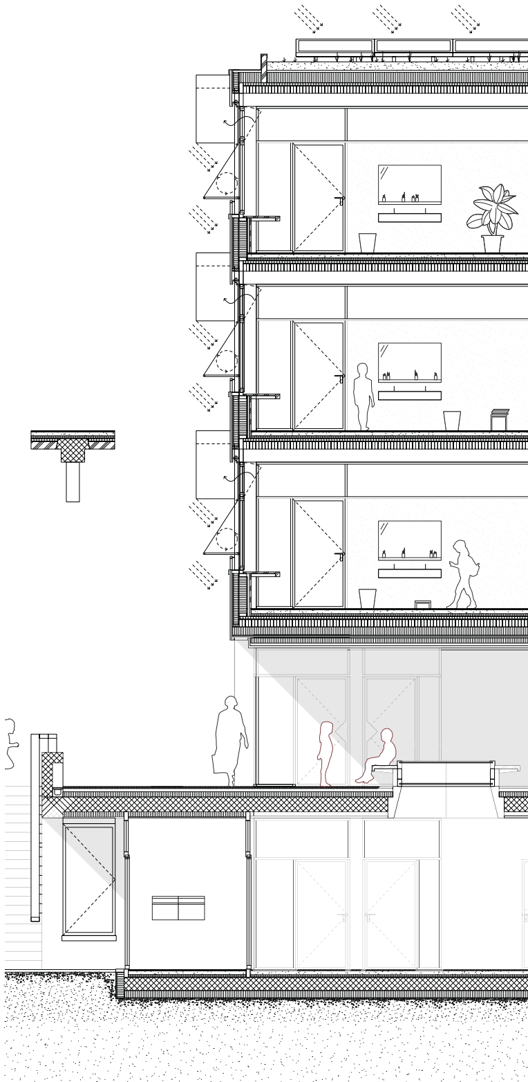
Konstruktionsschnitt und Ausschnitt Fassade 1:100
