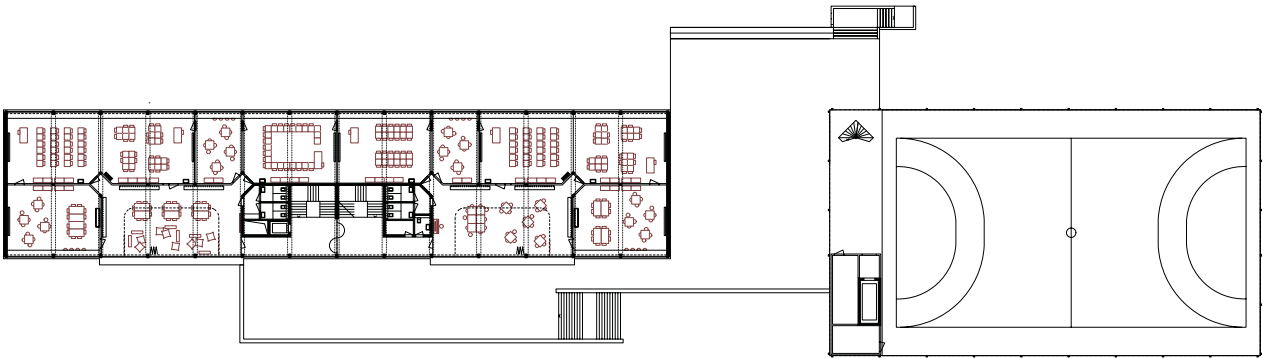
Grundriss 1.-3. Obergeschoss 1:800
