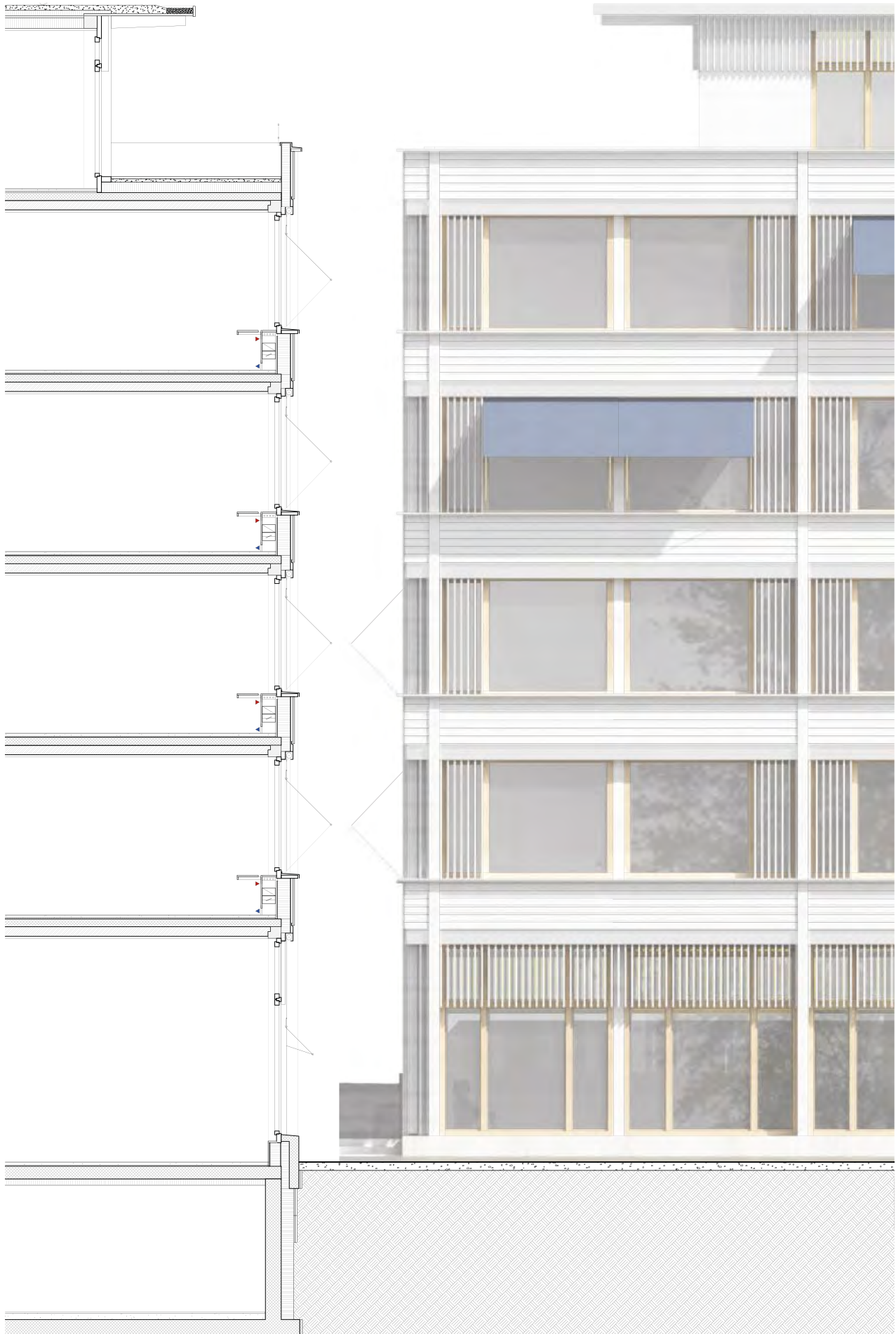
Konstruktionsschnitt und Ausschnitt Fassade 1:100
