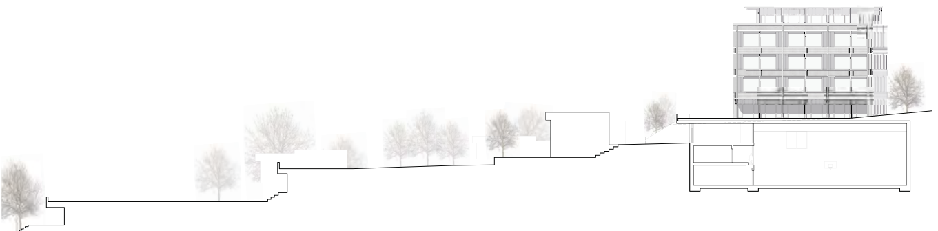
Ansicht Südost 1:800
