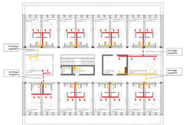
Lüftungskonzept 2. OG
