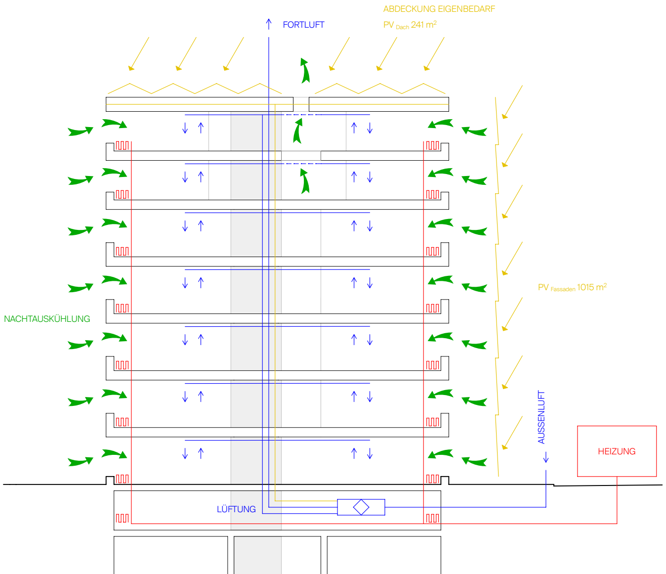
HAUSTECHNIK LOW-TECH
