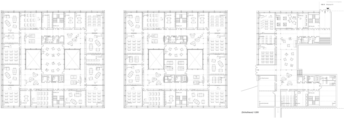
1., 2. Obergeschoss und Untergeschoss (Schulhaus)
