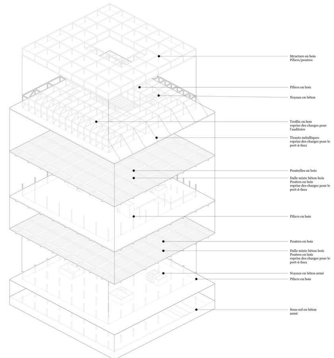
Axonometrie - principe statique
