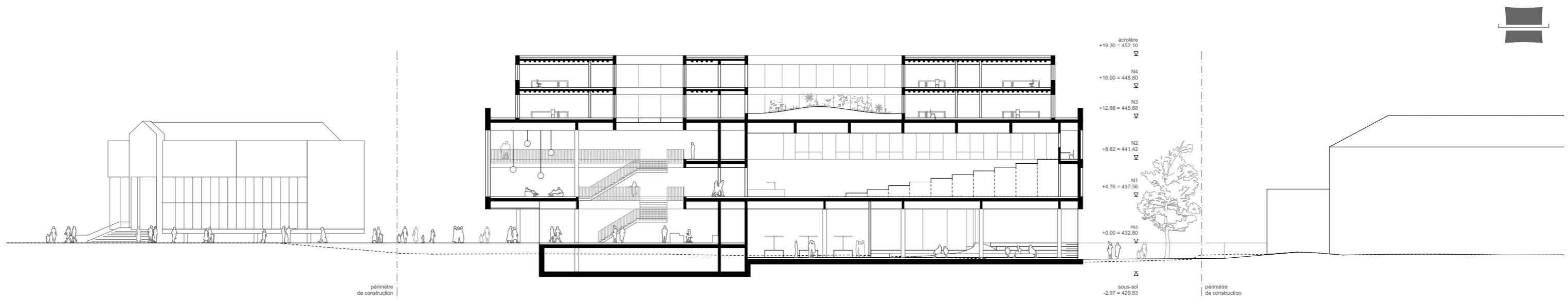
COUPE TRANSVERSALE 1 : 200
