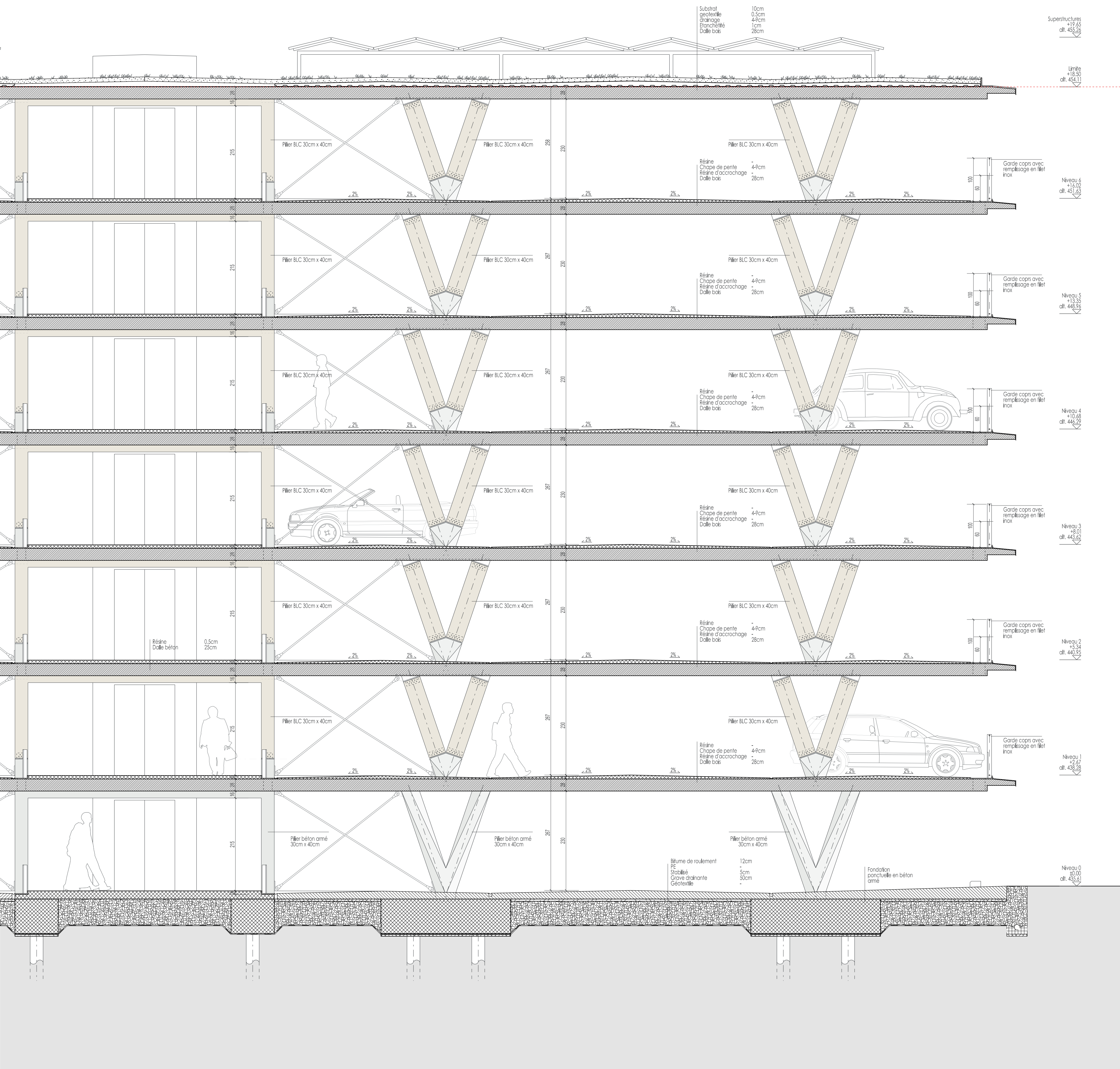
Coupe Constructive 1:50
