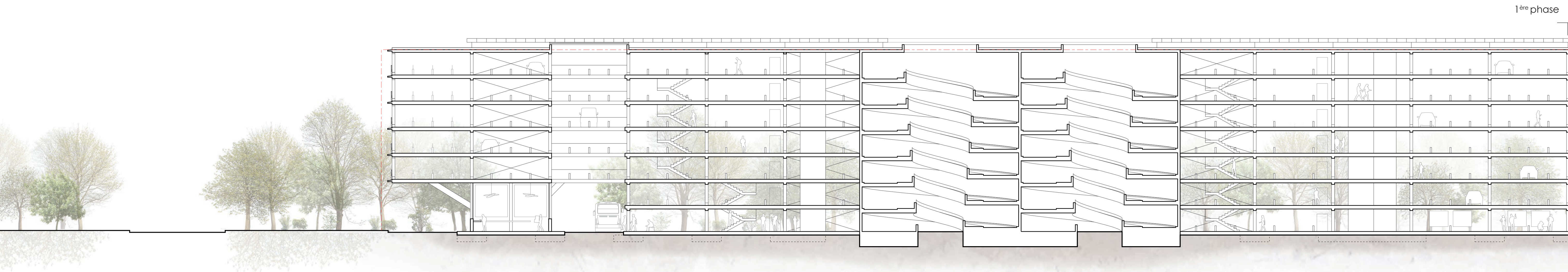
Coupe Longitudinale 1:200
