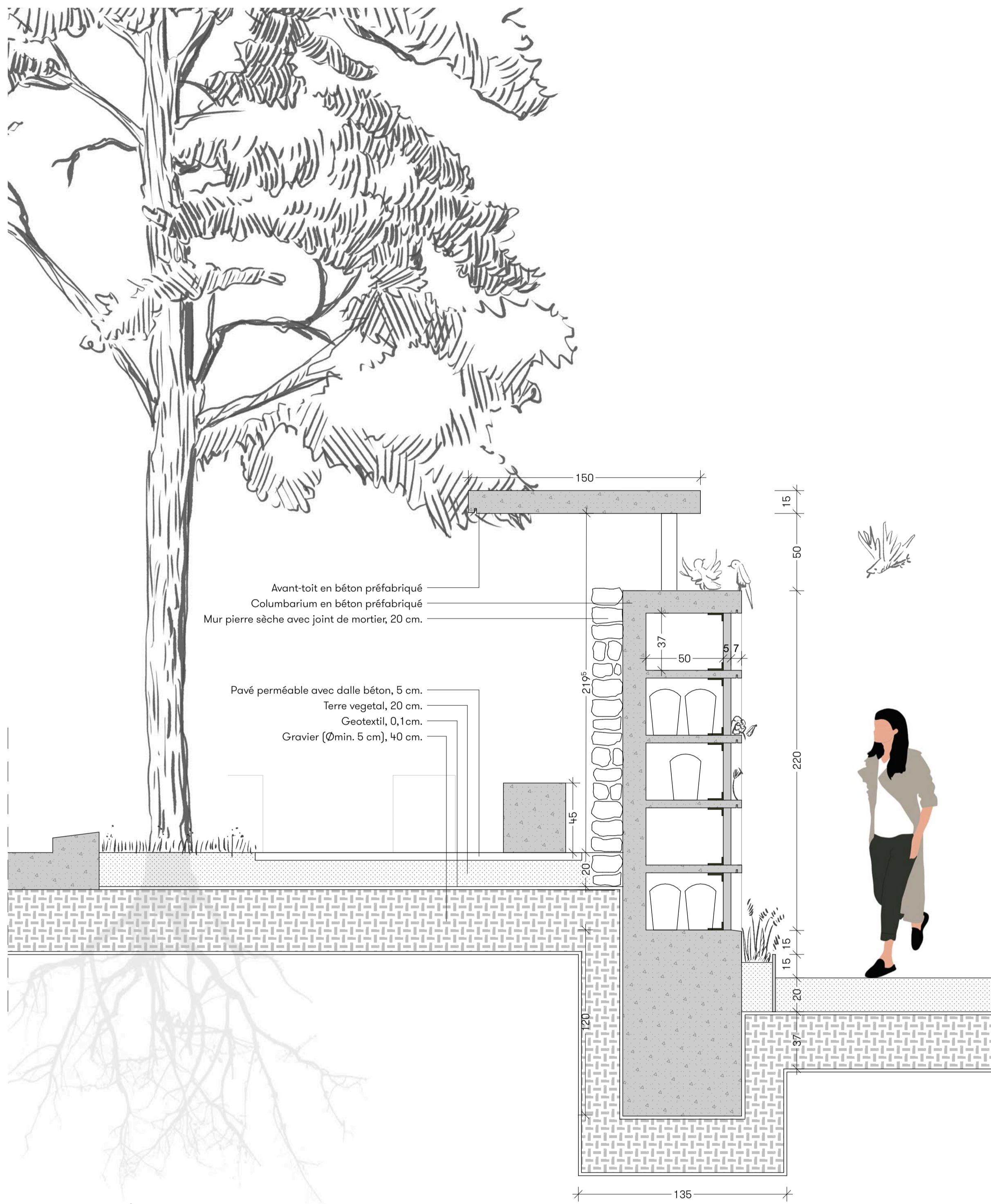
Détail Caveurnes 1/20
