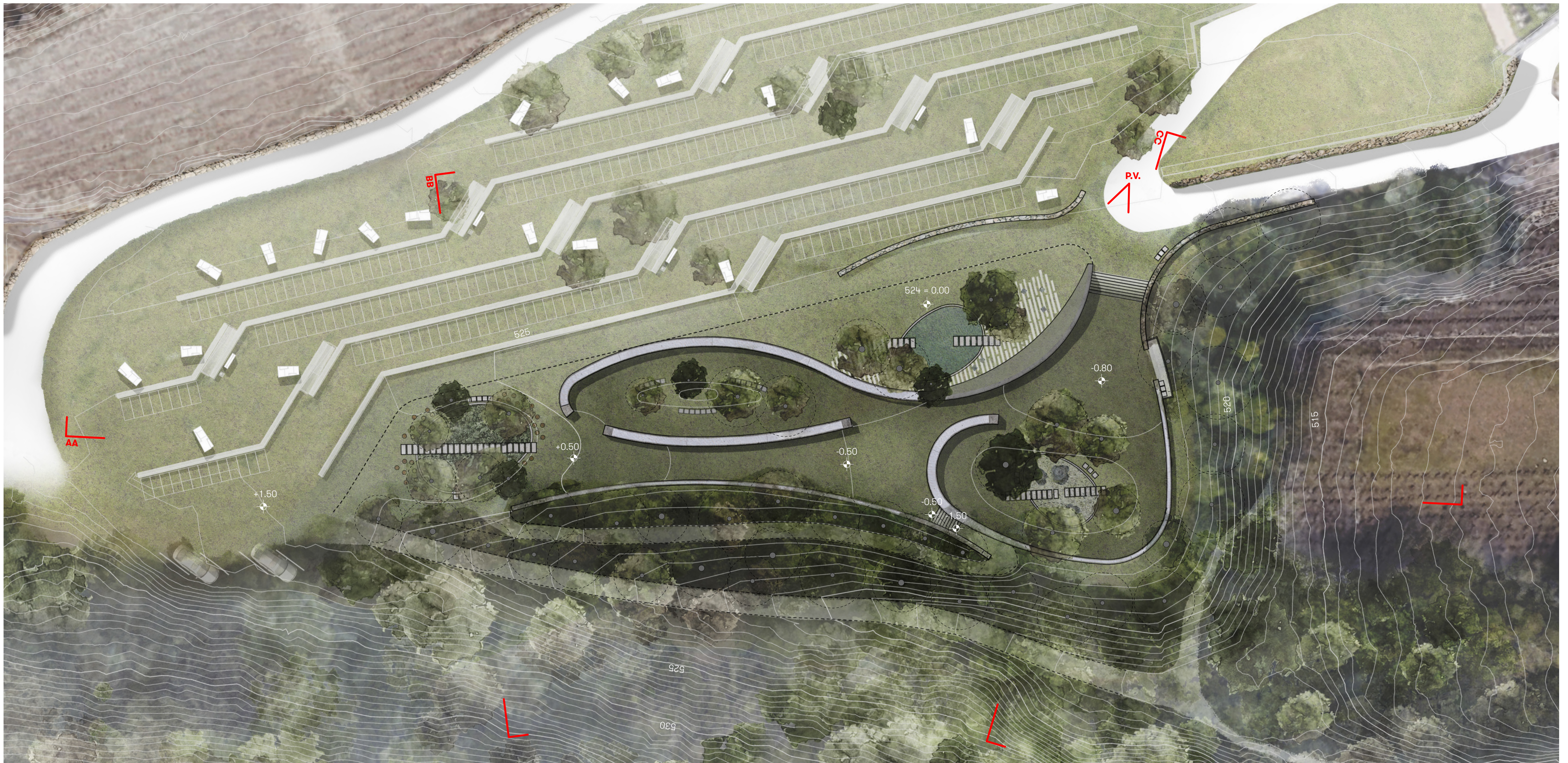
Plan de projet 1/200
