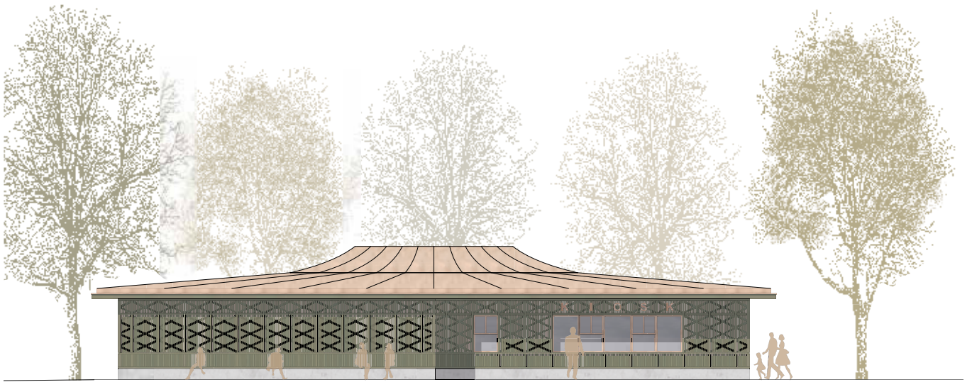
Ansicht West 1:200
