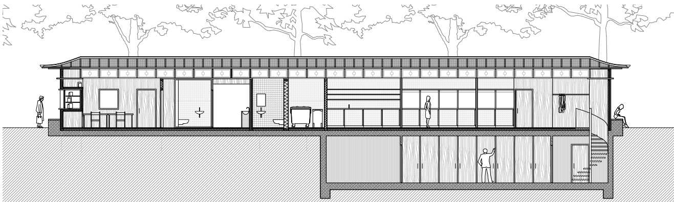
Längsschnitt 1:200
