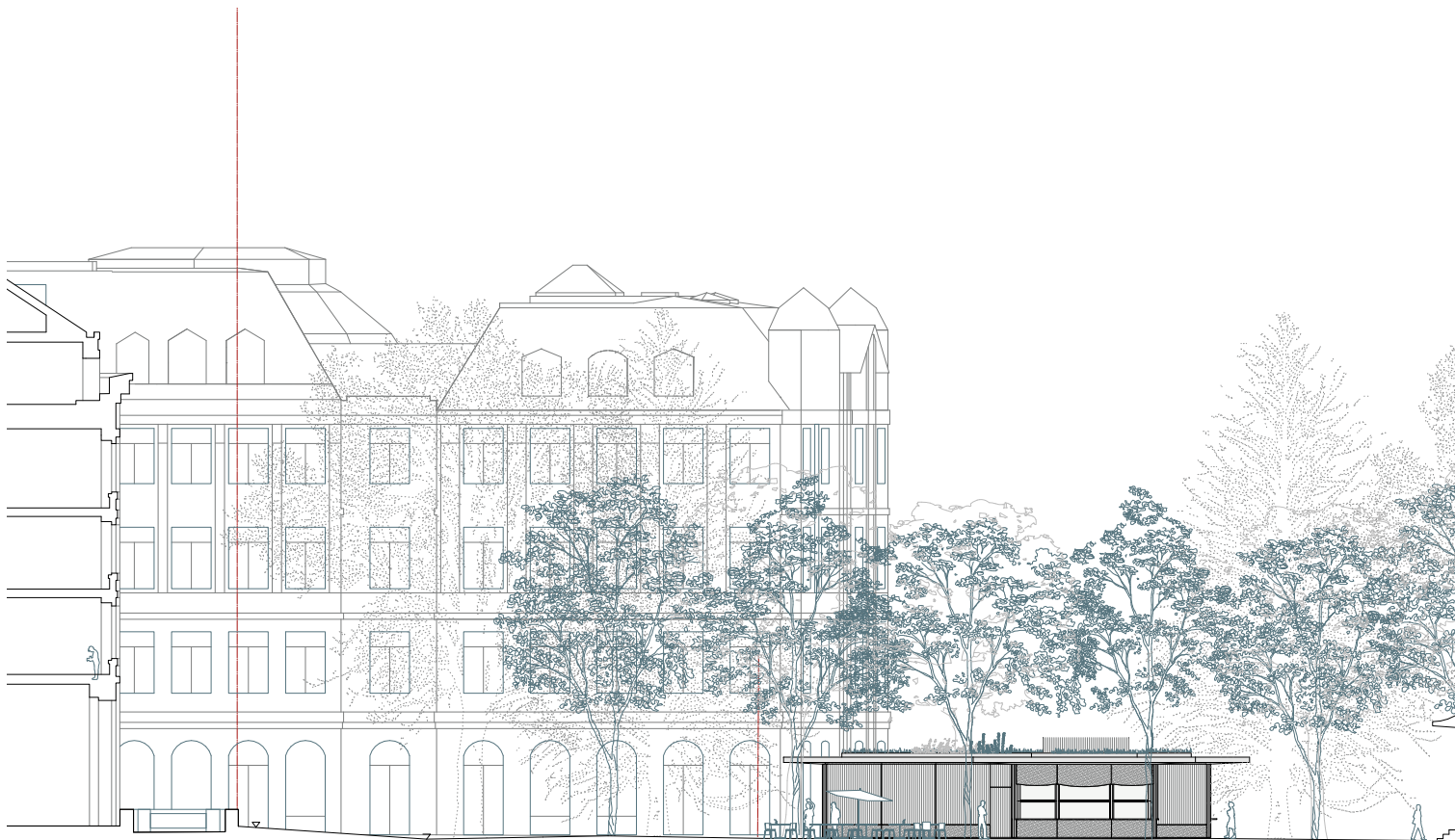
Längsschnitt Stadthausanlage 1:350
