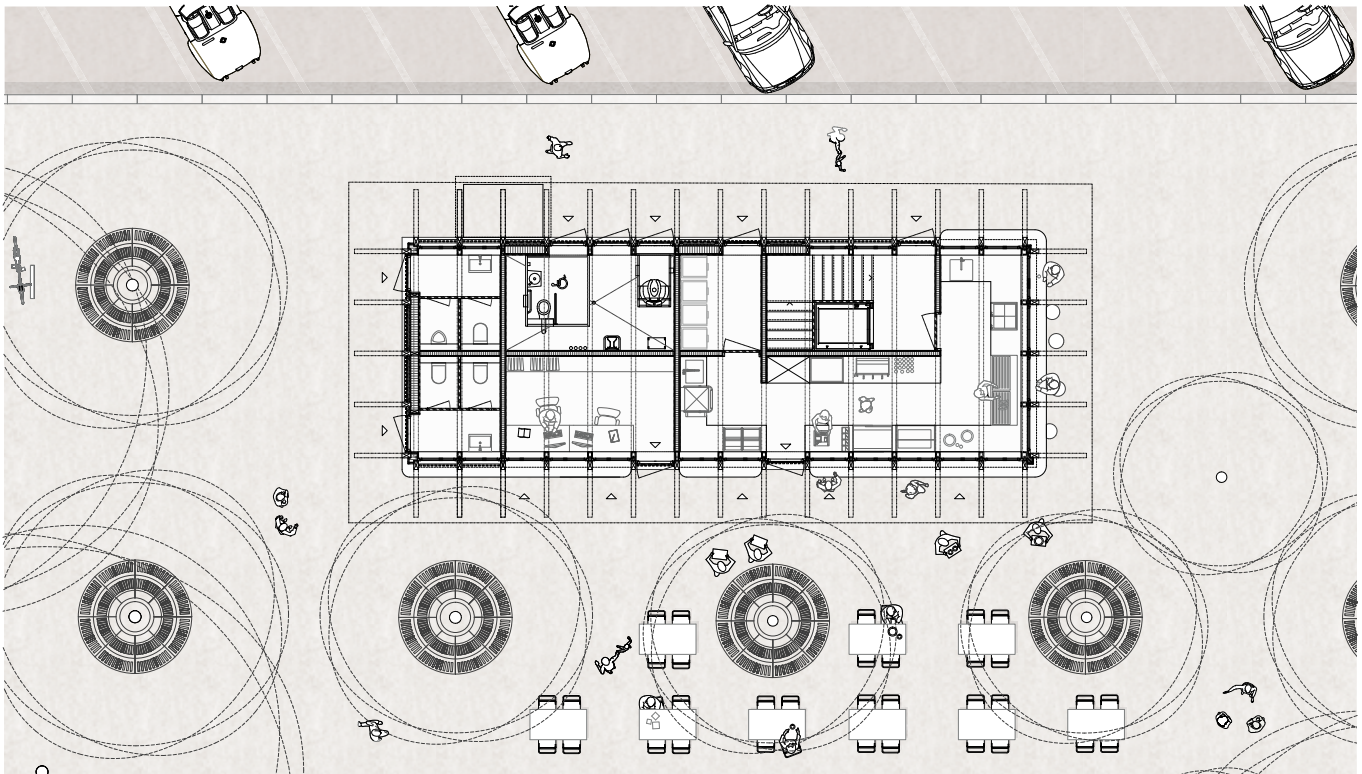
Grundriss Erdgeschoss 1:200
