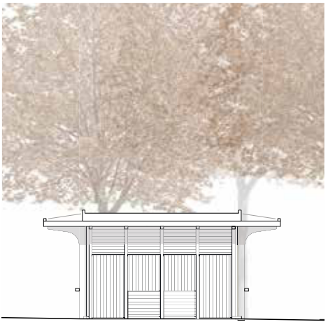
Ansicht Nord 1:200
