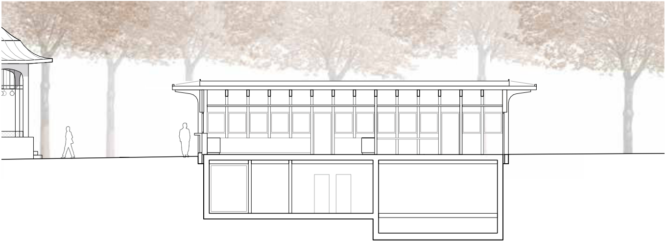
Längsschnitt 1:200
