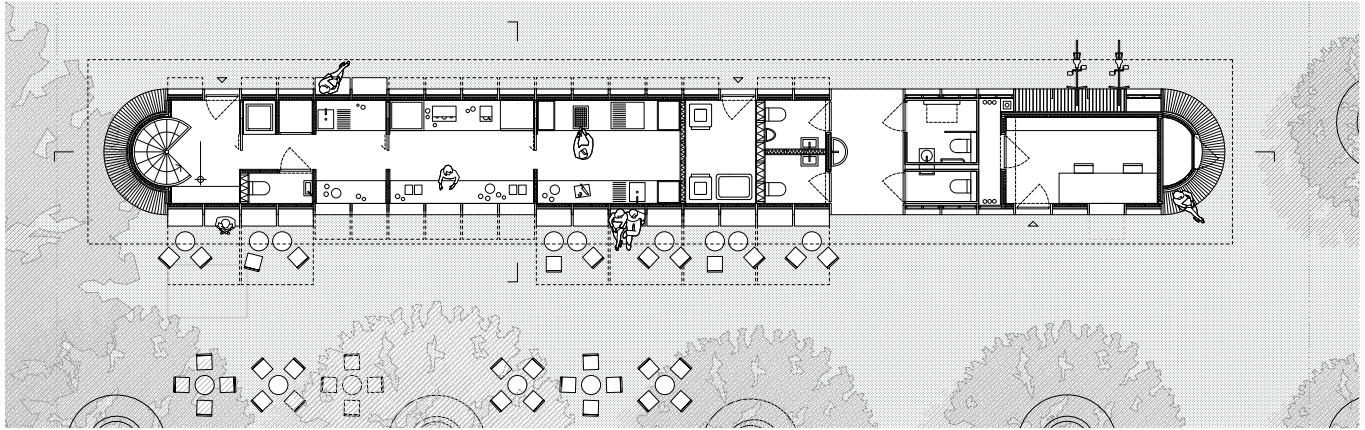
Grundriss Erdgeschoss 1:200
