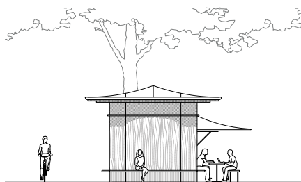
Ansicht Nord 1:200
