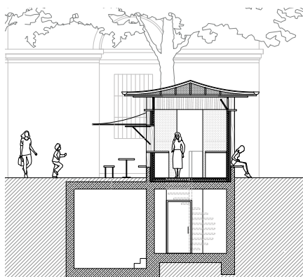
Querschnitt 1:200
