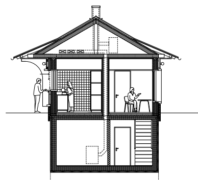
Querschnitt 1:200
