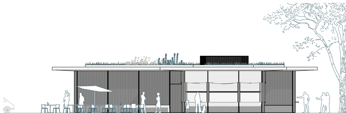
Ansicht West 1:200
