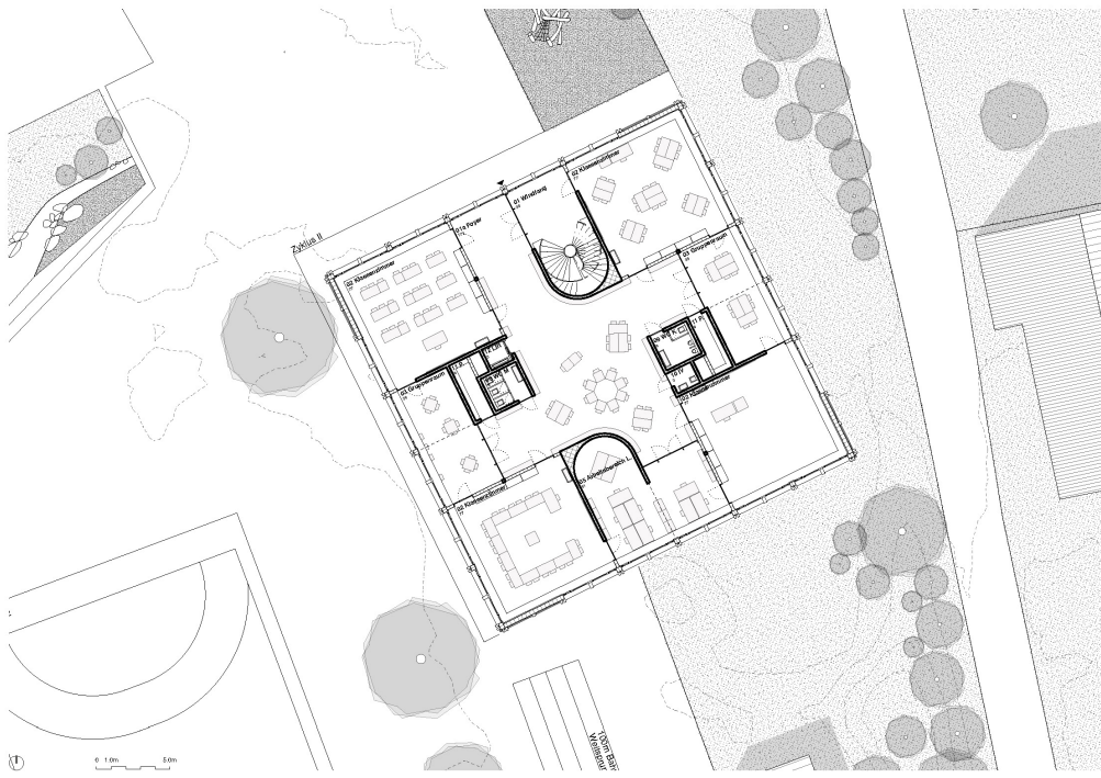
Grundriss 1 Obergeschoss 1:200
