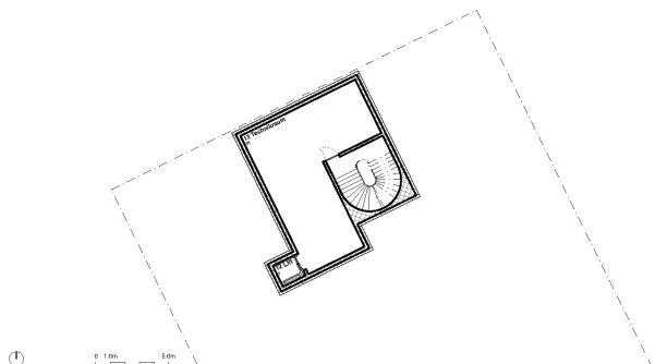
Grundriss Untergeschoss 1:200
