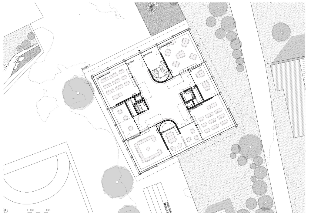
Grundriss 2 Obergeschoss 1:200
