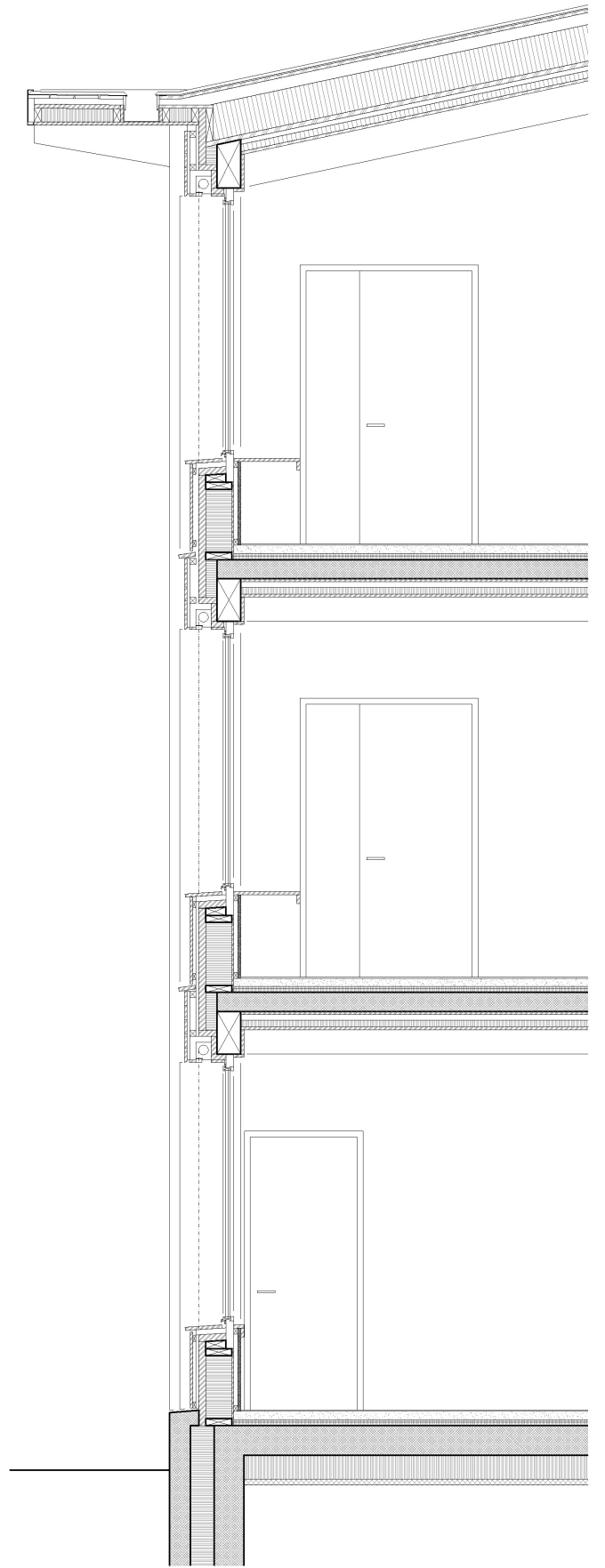
Detailansicht, Schulhaus 1:20
