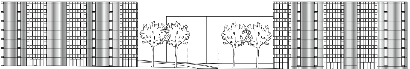
Strassenansicht Westbereich 1:750
