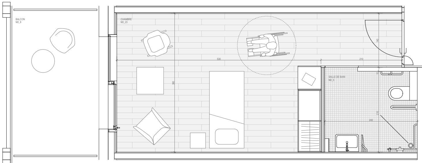
PLAN CHAMBRE 1/20
