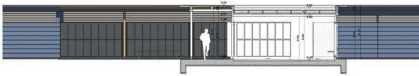
Fassadenschnitt Garderobe neu Mst. 1:50 (verkleinert)
