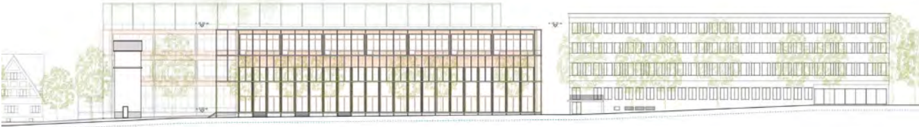
Südwestansicht
