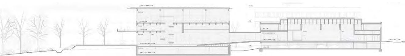
Bibliotheksgebäude, Schnitt
