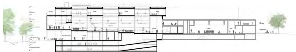
Schnitt A-A
