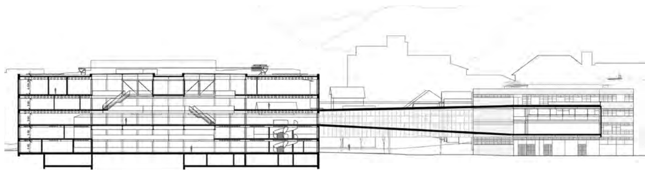
Schnitt Nordost-Südwest
