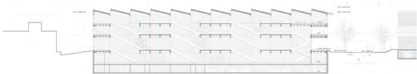
Hauptgebäude, Schnitt
