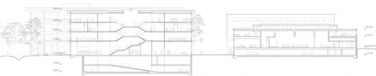
Querschnitt C-C
