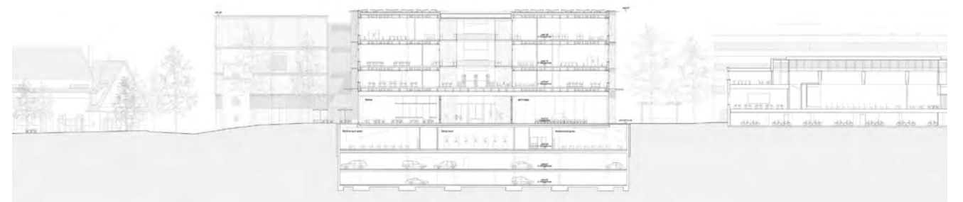
Querschnitt Südgebäude
