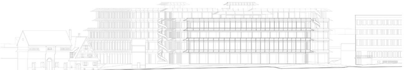
Ansicht Süd
