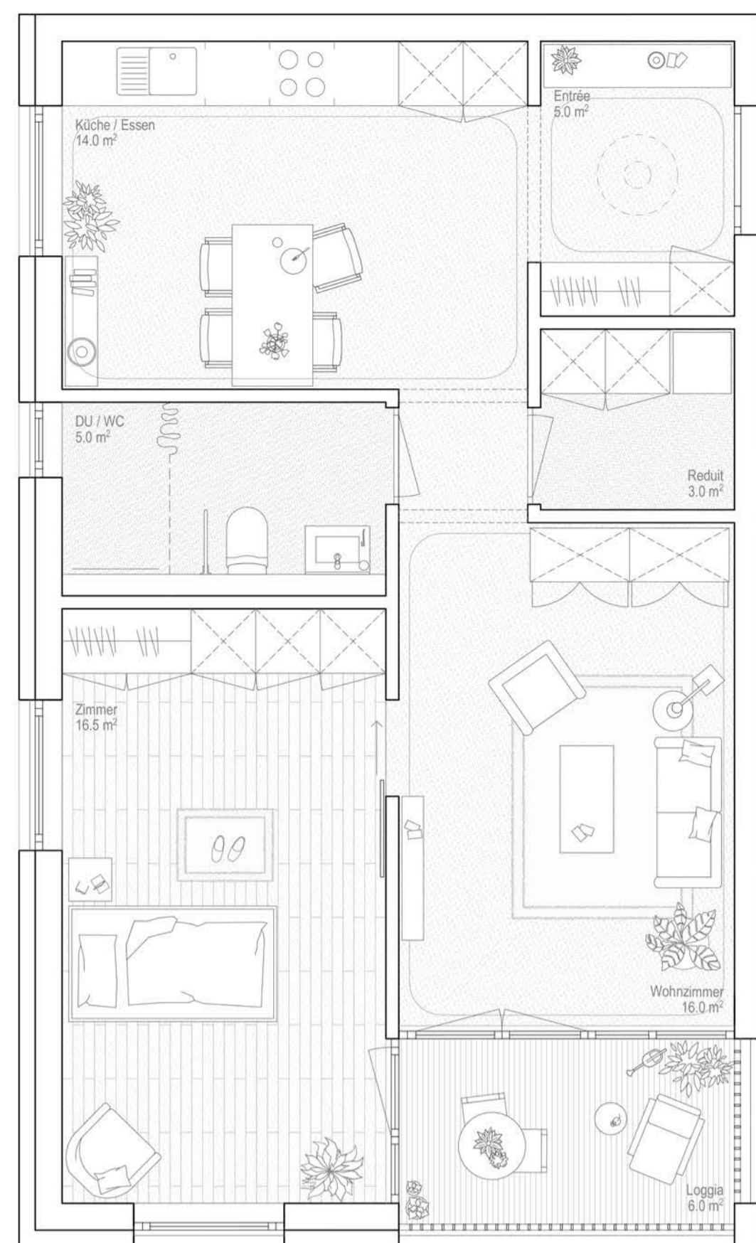
Typ 2.5-Zi-Wohnung 59.5m²
