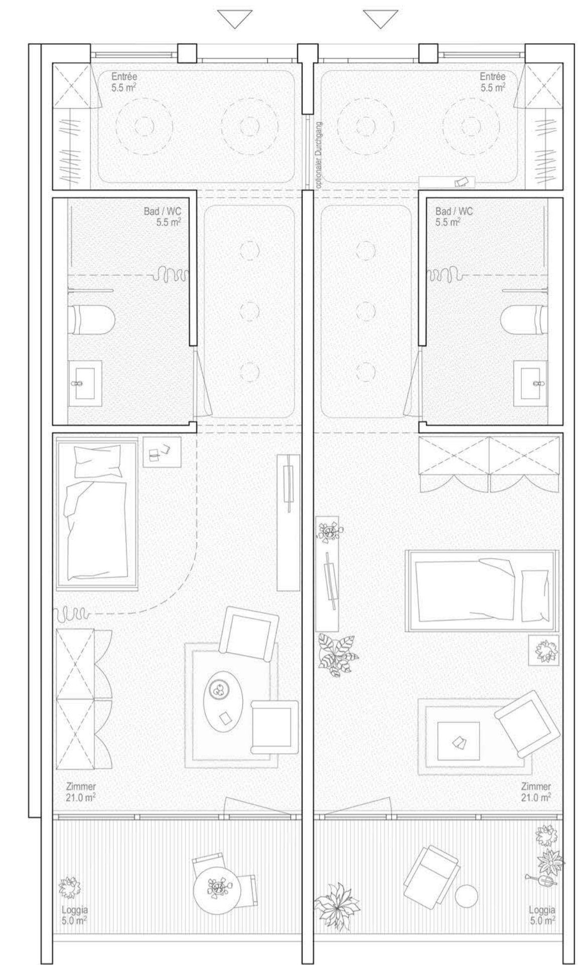
Typ Pflegezimmer 2. OG Bestand 32.0m²
