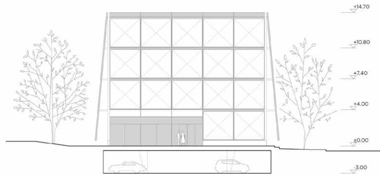
OSTFASSADE
