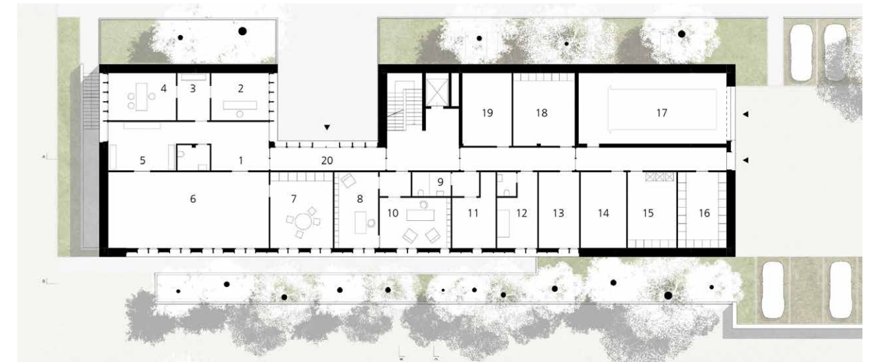
Erdgeschoss + 0.20
