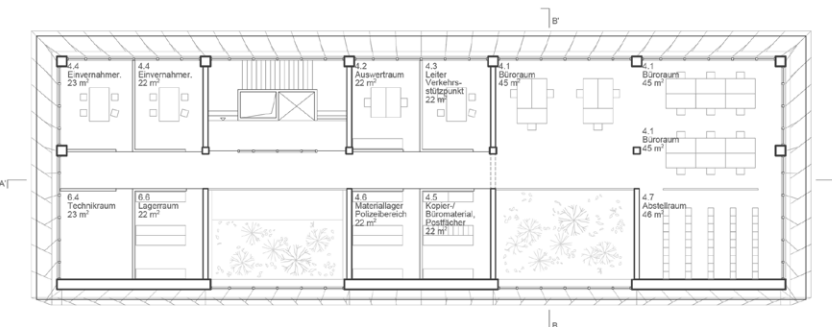
Grundriss 2. Obergeschoss 1:200
