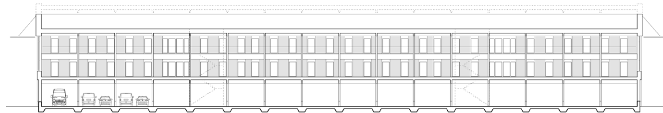
Längsschnitt M 1:250
