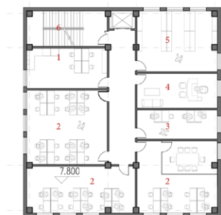
2.Obergeschoss Eingang 1:200
