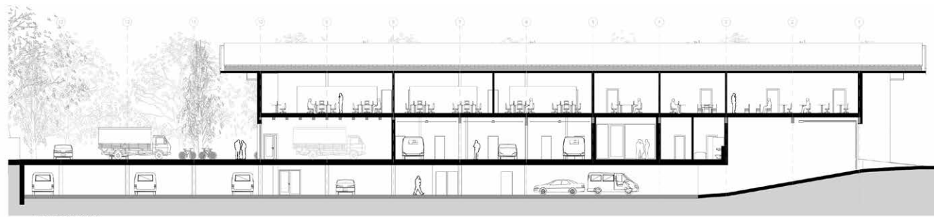
Längsschnitt 1:200
