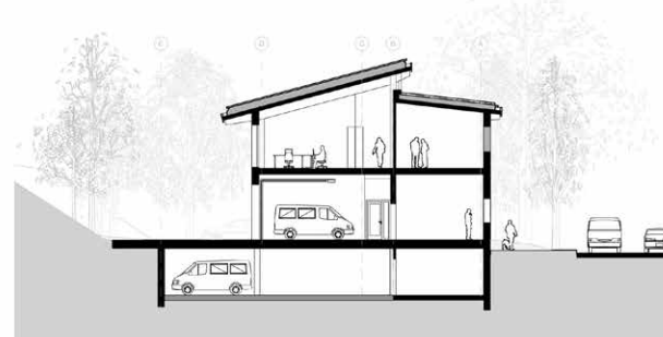
Querschnitt 2 - 1:200
