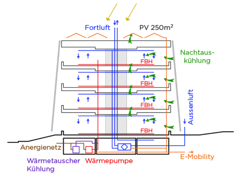
HAUSTECHNIK LOW-TECH
