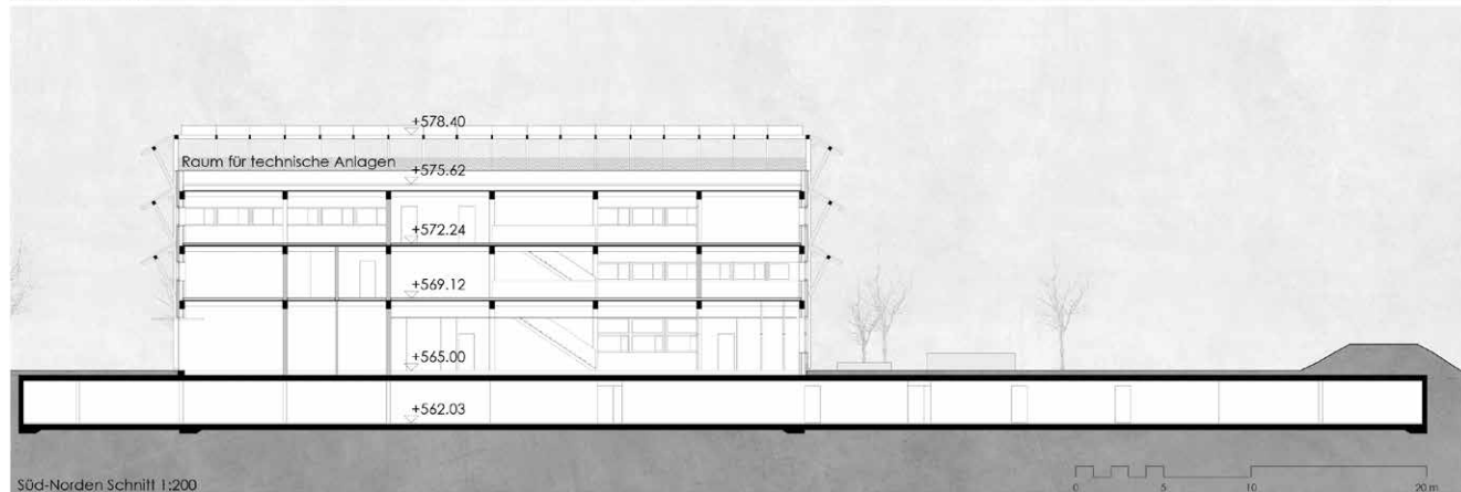
Süd-Norden Schnitt 1:200
