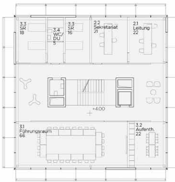
1. OG
