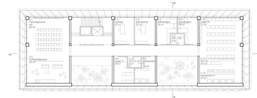
Grundriss 1. Obergeschoss 1:200
