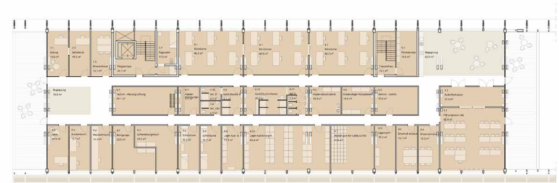
Obergeschoss M 1:200
