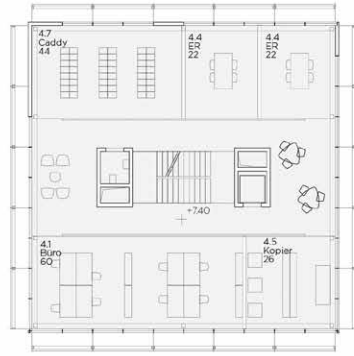
2. OG
