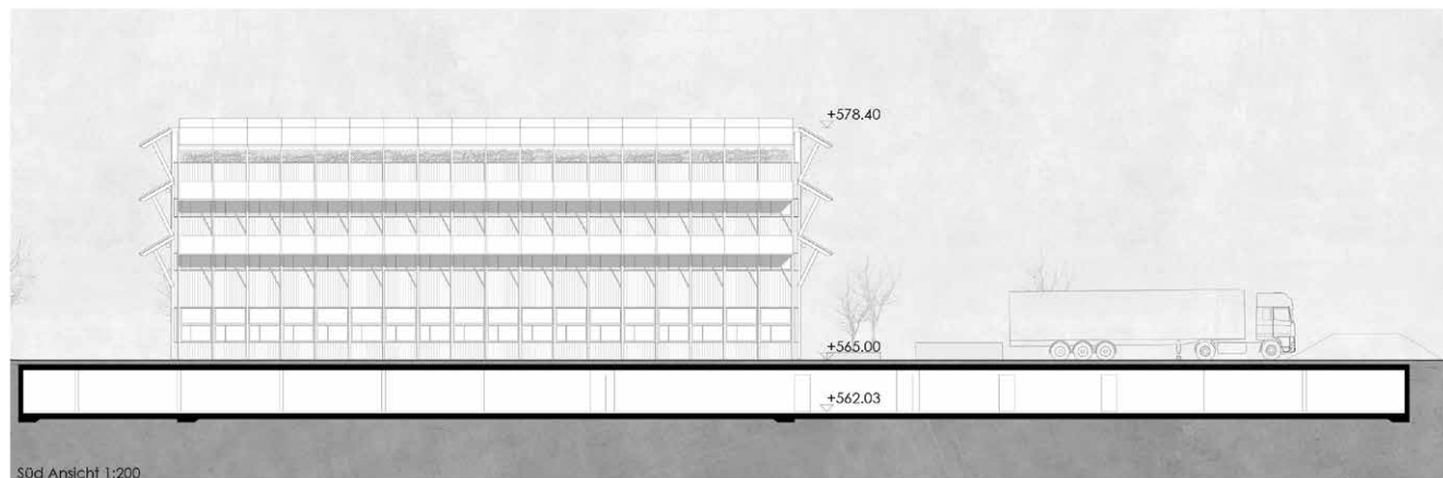
Süd Ansicht 1:200
