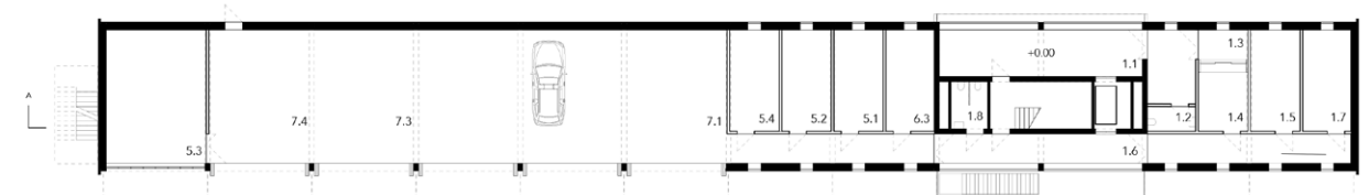
Erdgeschoss 1:200
