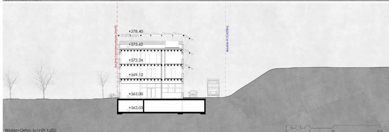
Westen-Osten Schnitt 1:200
