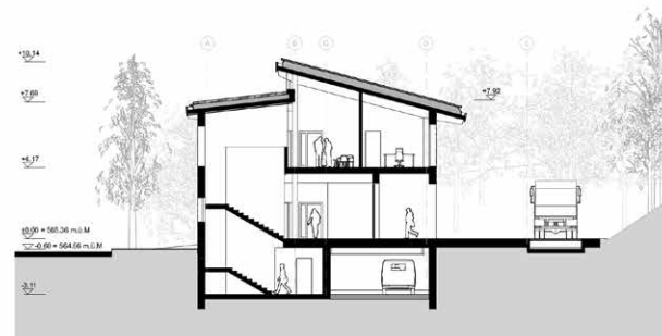
Querschnitt 1 - 1:200
