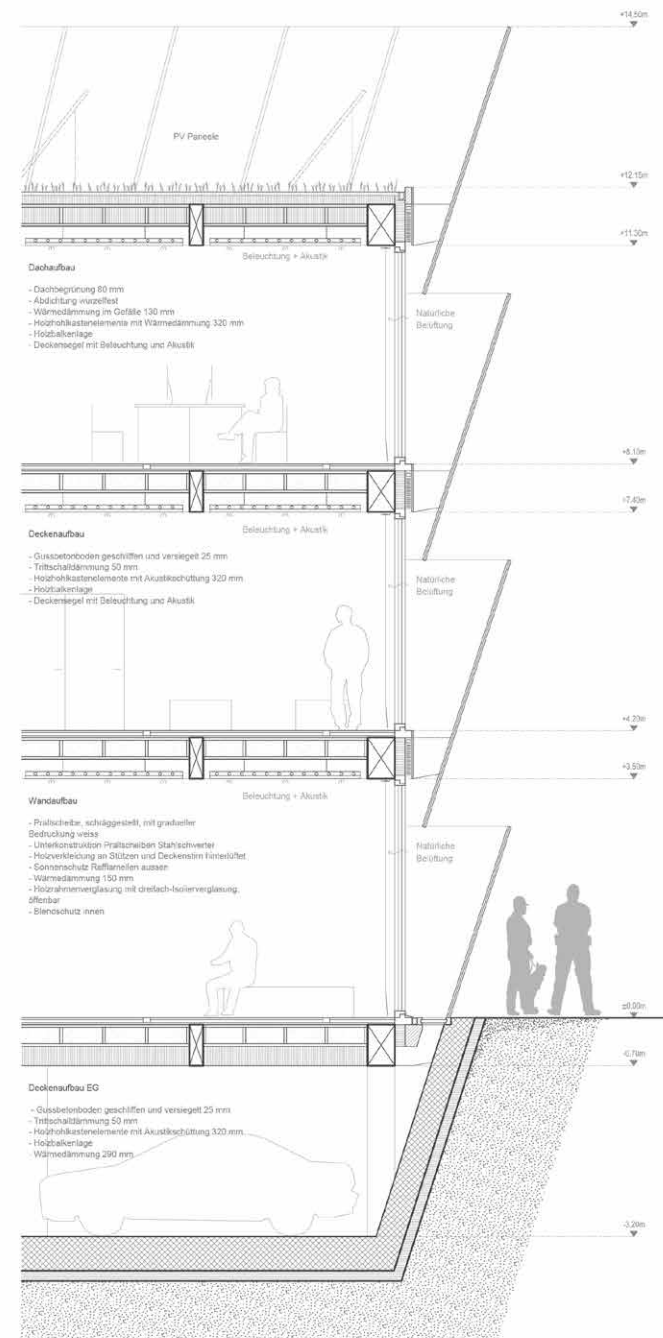
Fassadendetail 1:50
