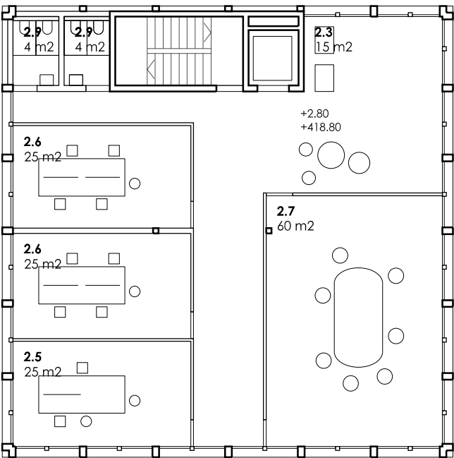
Plan rez supérieur - 1/200
