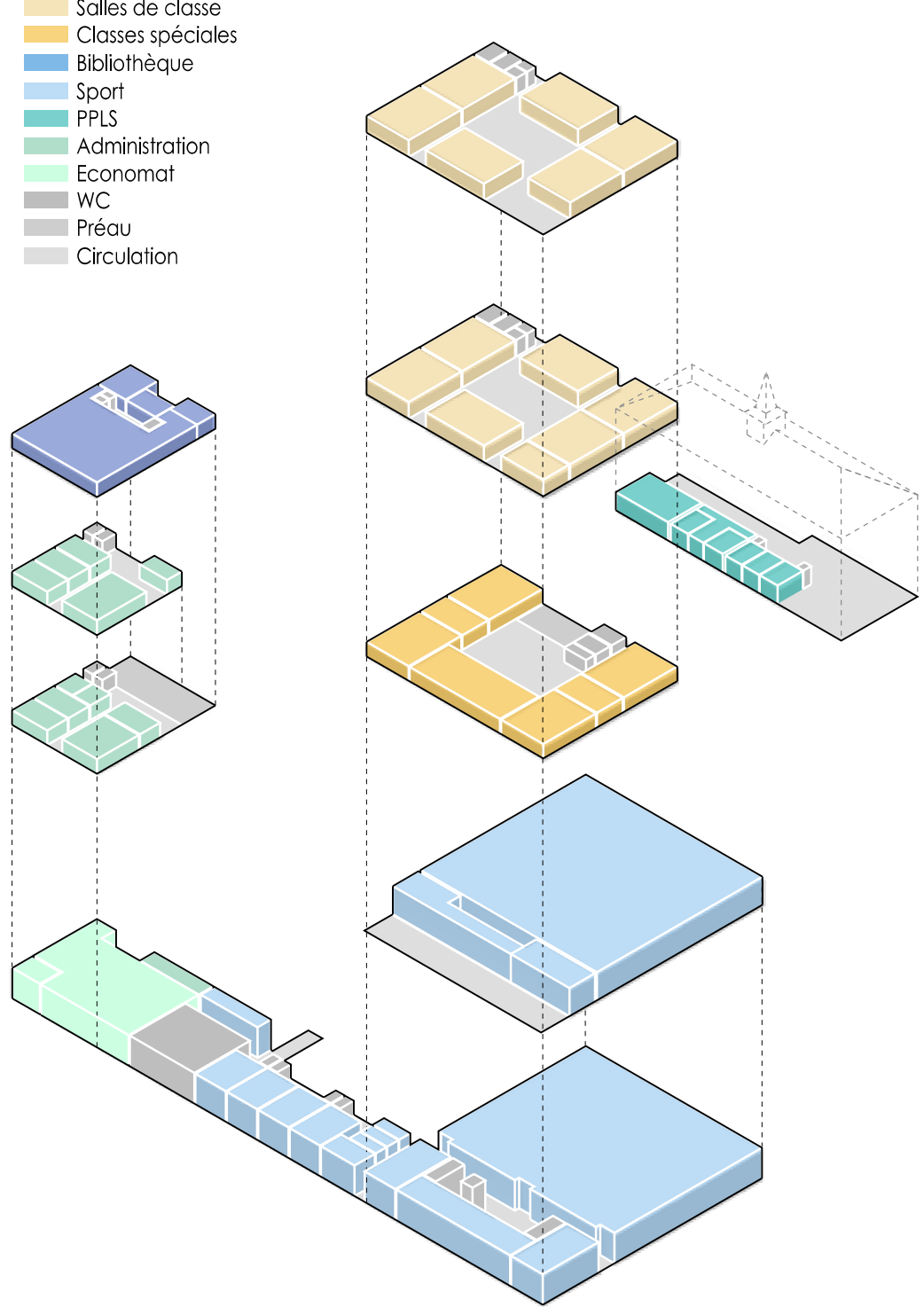
Axonométrie du programme
