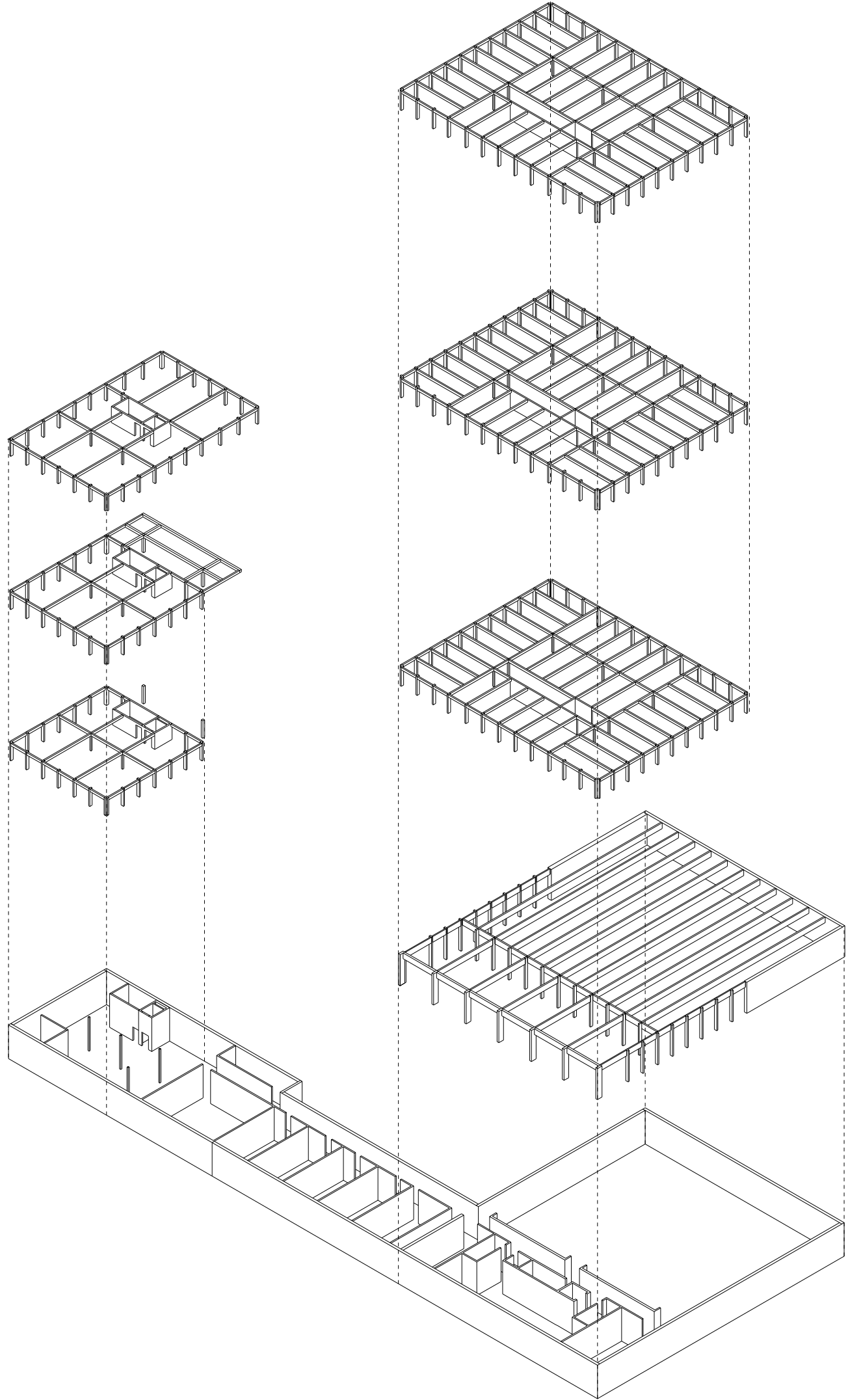
Schéma structurel
