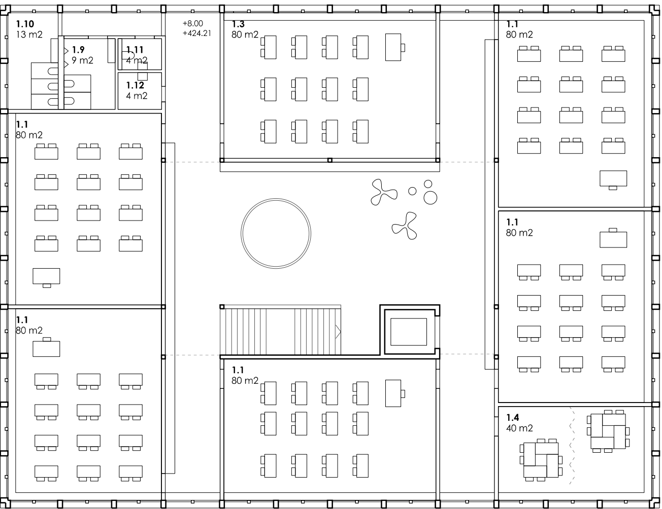
Plan R+2 - 1/200
