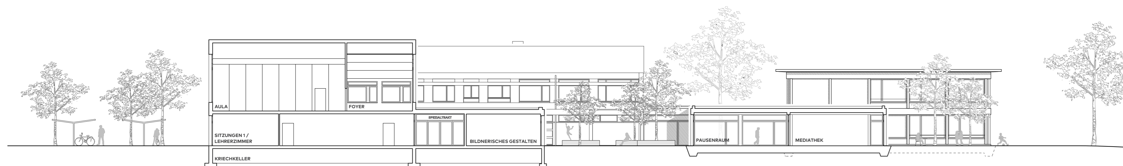
Fassadenansicht Südwest mit Hof | 1:200
