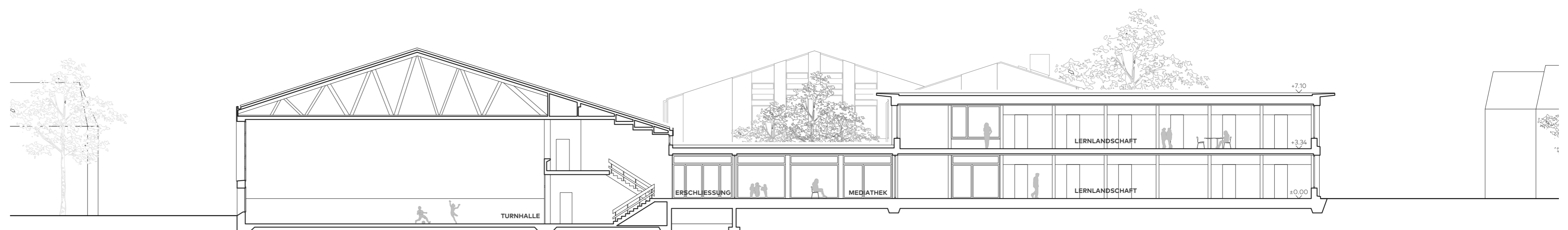
Längsschnitt B-B | 1:200
