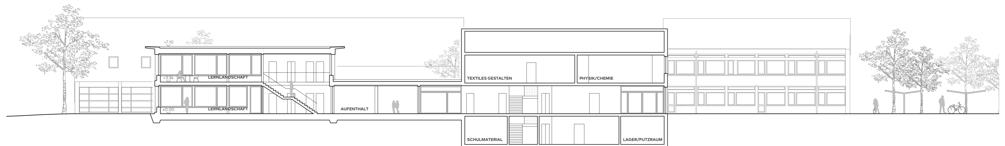
Querschnitt A-A | 1:200
