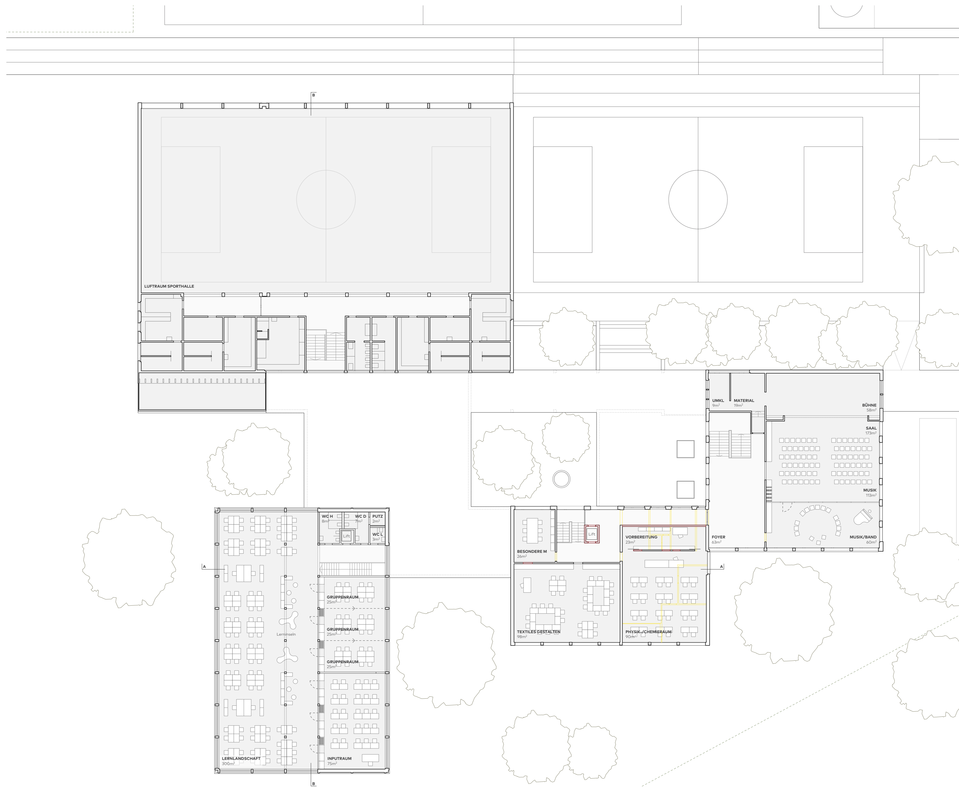
Obergeschoss | 1:200
