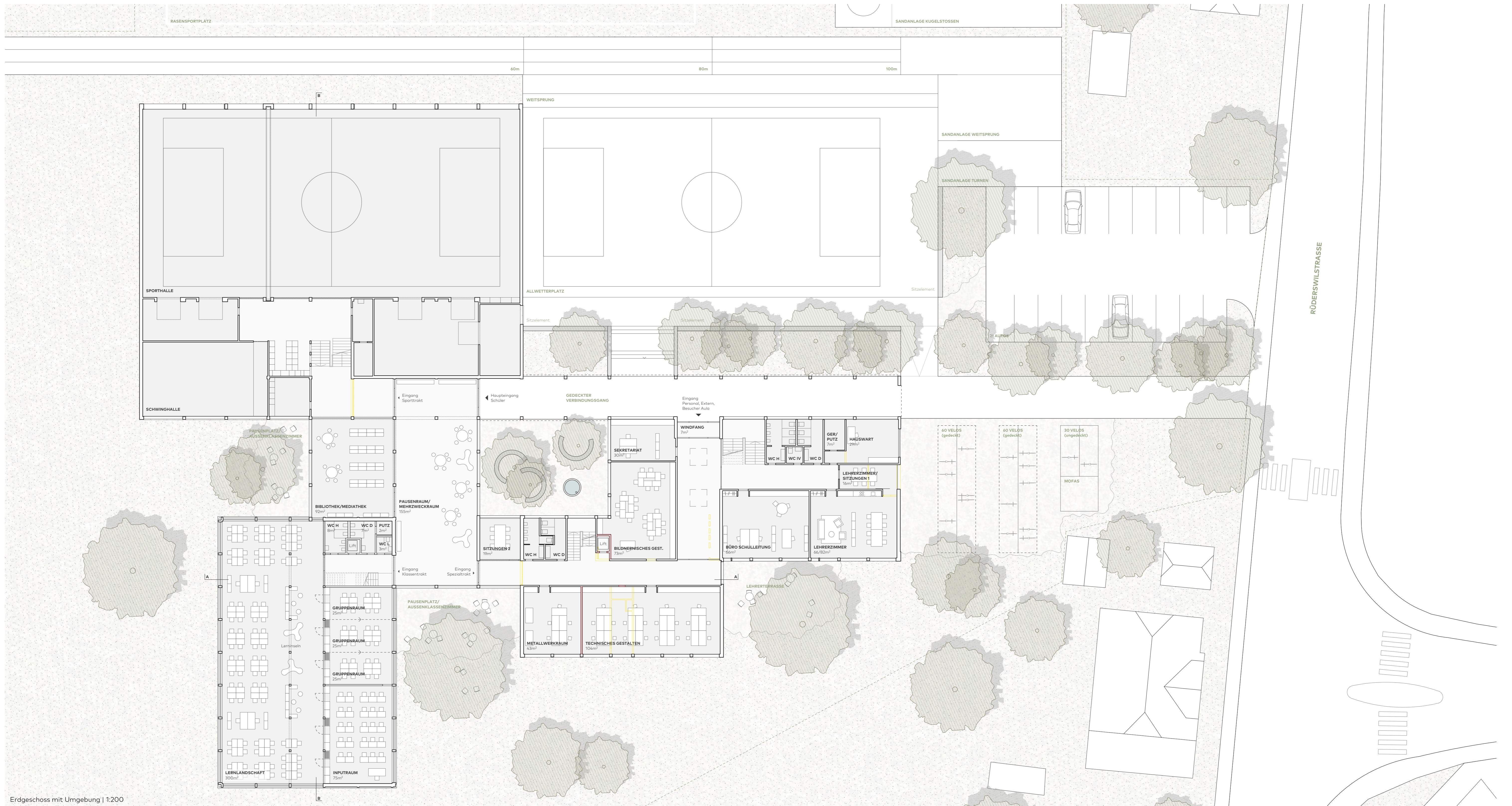
Erdgeschoss mit Umgebung | 1:200
