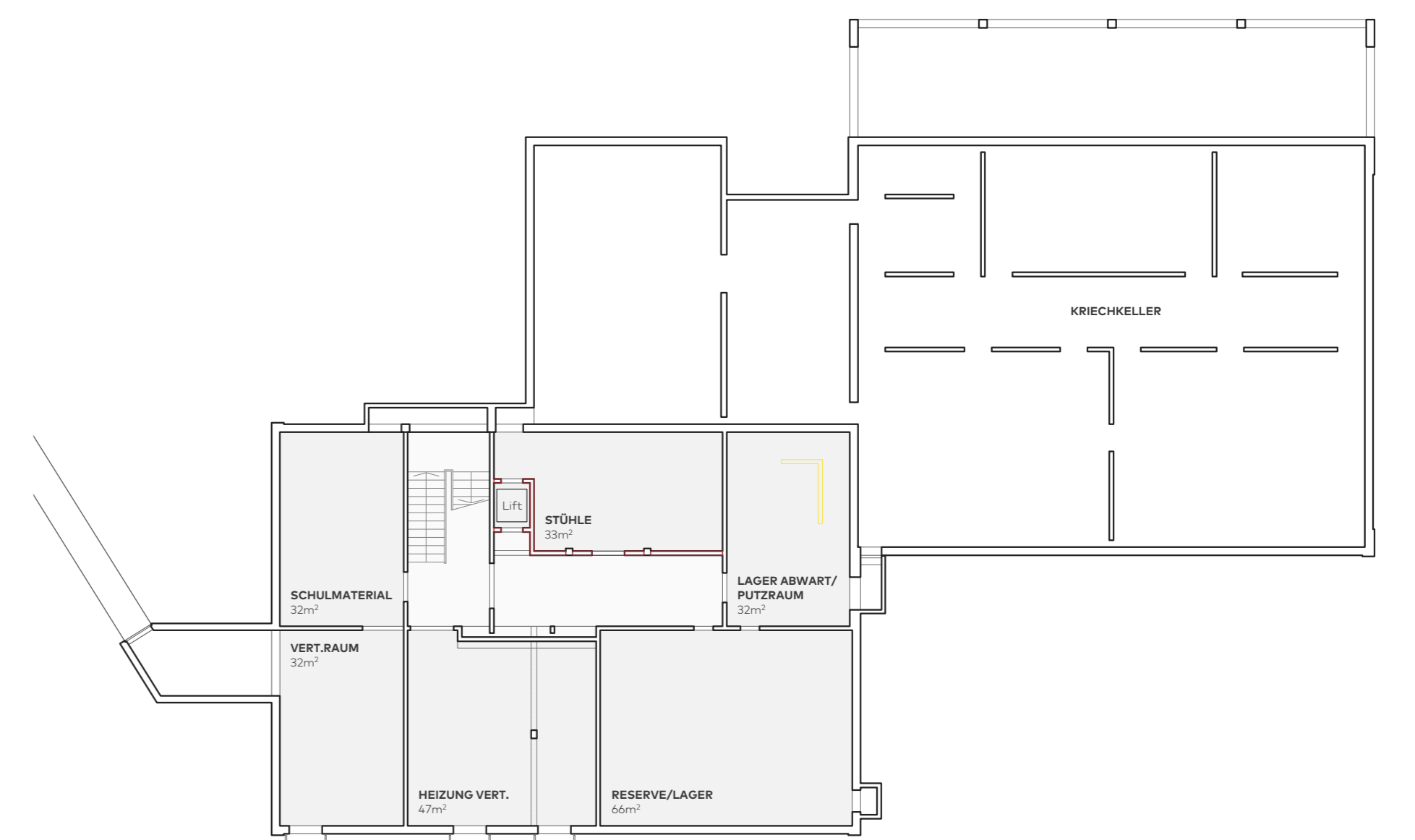
Untergeschoss | 1:500
