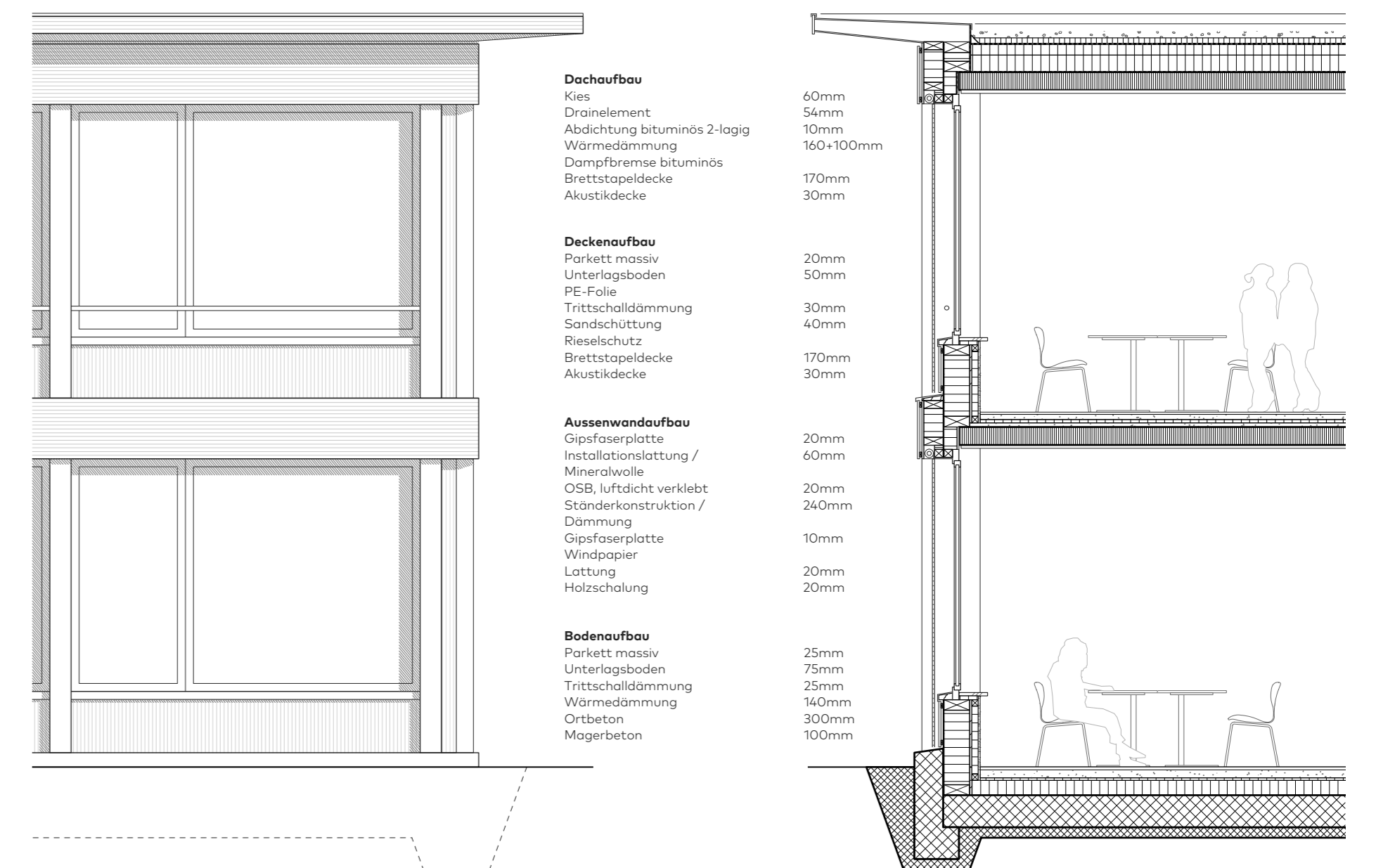
Fassadenschnitt | 1:50
