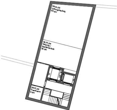
3. Untergeschoss
