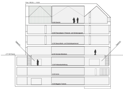
Längsschnitt (Ost-West)
