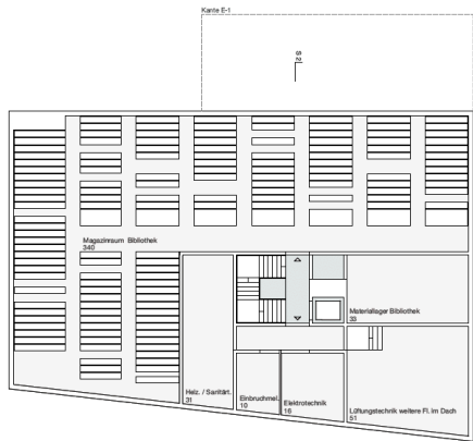
3. Untergeschoss
