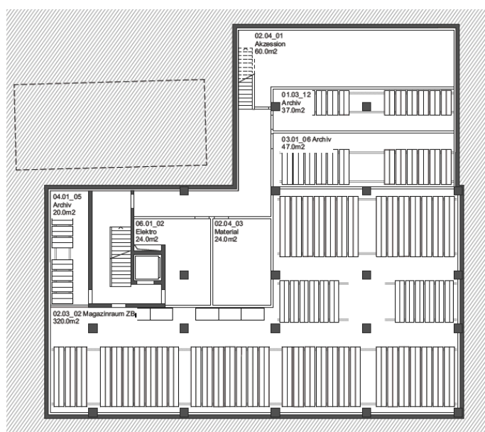
2. Untergeschoss
