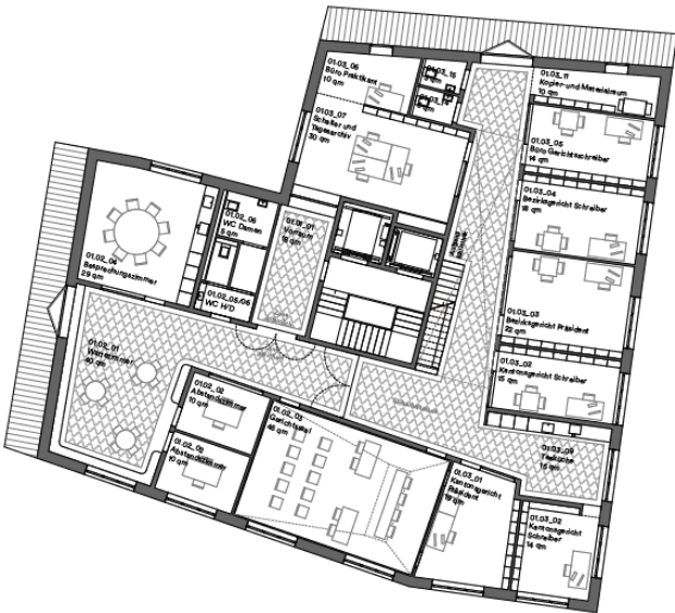
3. Obergeschoss
