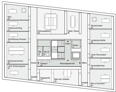
2. Obergeschoss
