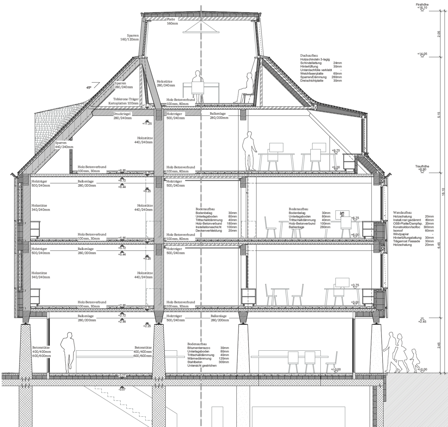
Fassadenschnitt
