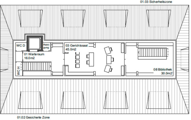
2. Dachgeschoss
