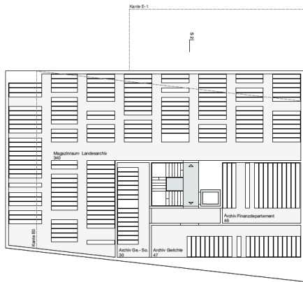
2. Untergeschoss
