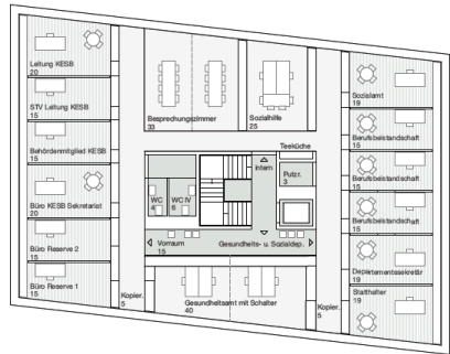
1. Obergeschoss
