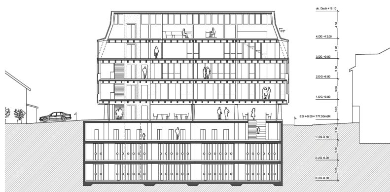
Längsschnitt (Ost-West)
