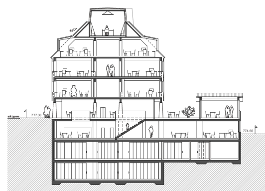
Querschnitt (Nord-Süd)
