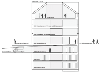
Querschnitt (Nord-Süd)
