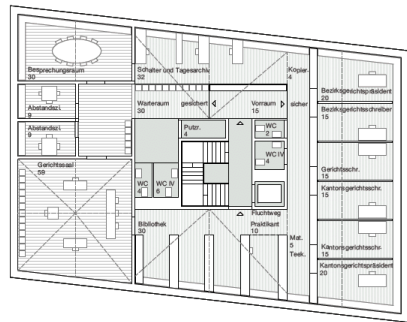
3. Obergeschoss
