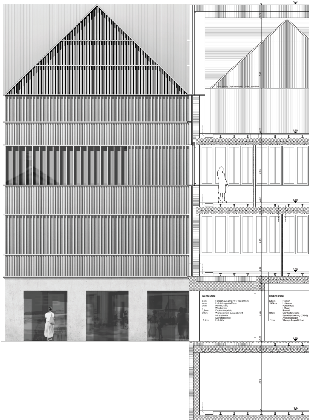
Fassadenschnitt
