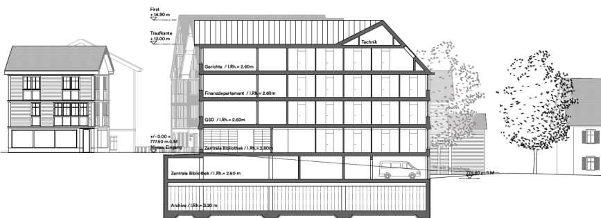
Längsschnitt (Nord-Süd)
