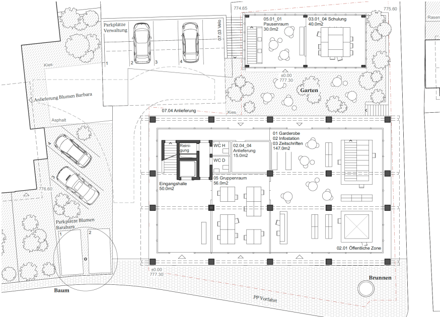
Erdgeschoss
