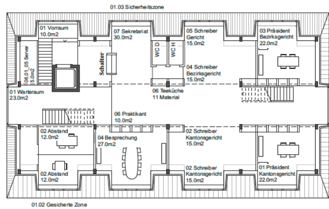
1. Dachgeschoss
