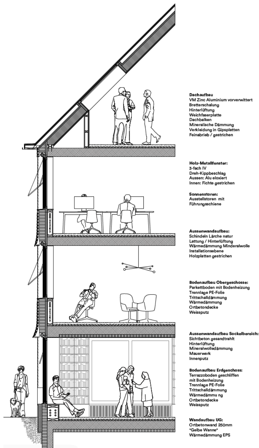
Fassadenschnitt
