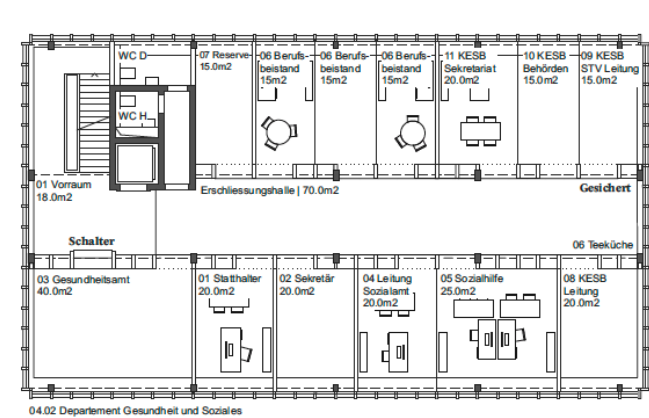
1. Obergeschoss
