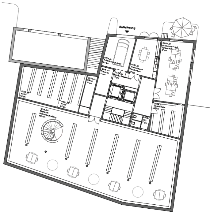
1. Untergeschoss
