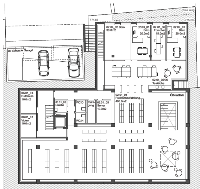
1. Untergeschoss
