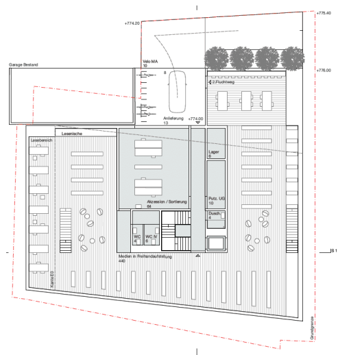
1. Untergeschoss
