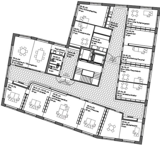
2. Obergeschoss
