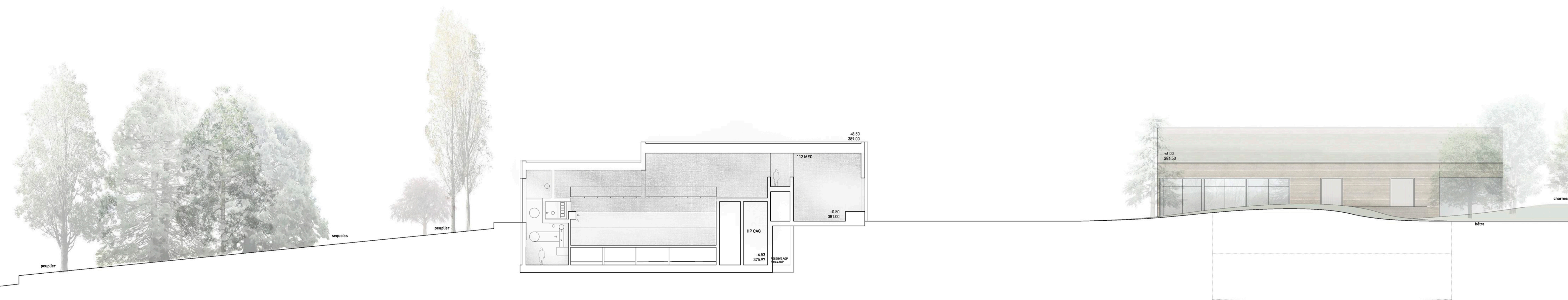
COUPE E 1:200 0 5
