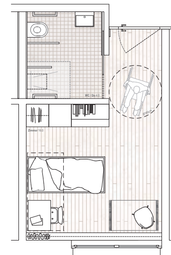
Pflegezimmer Langzeitpflege 1:100
