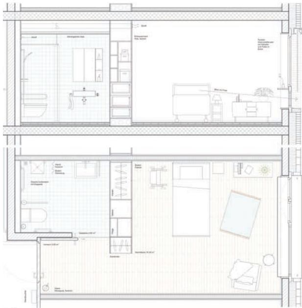
Pflegezimmer 1:100
