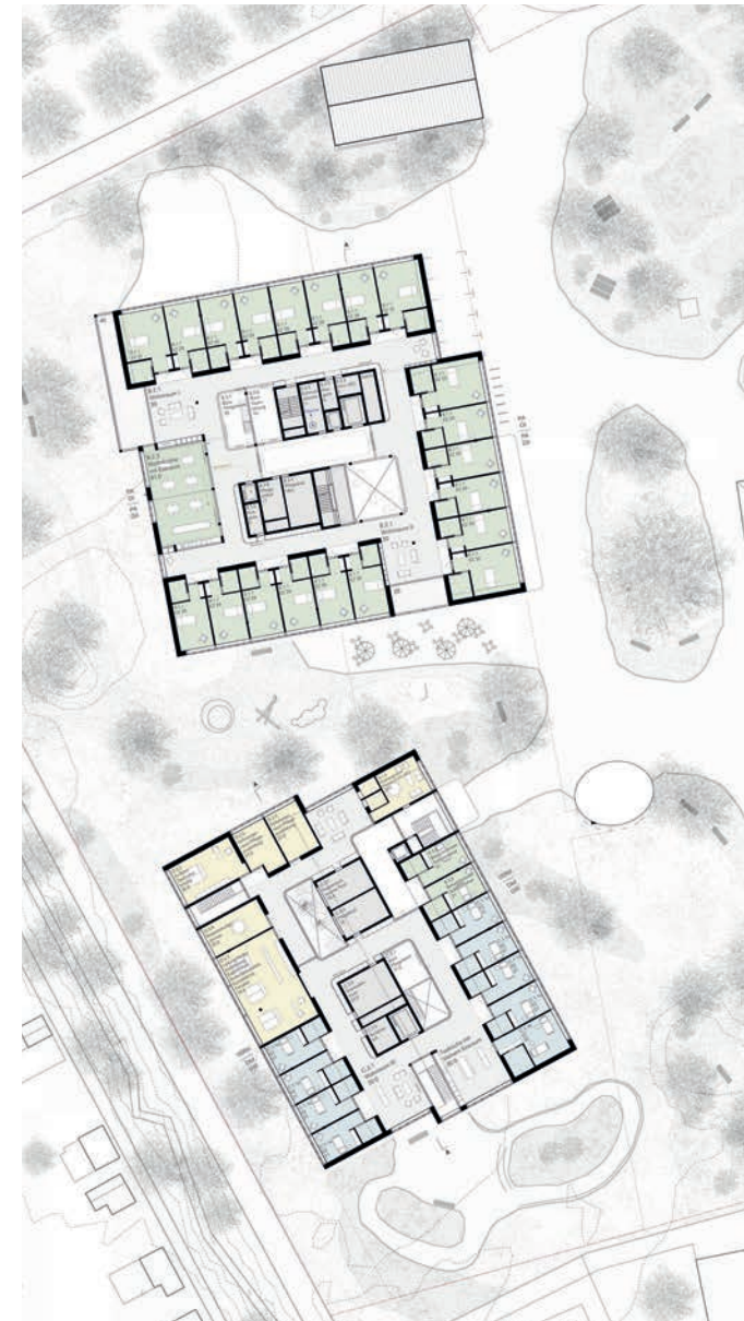
1. Obergeschoss 1:1000
