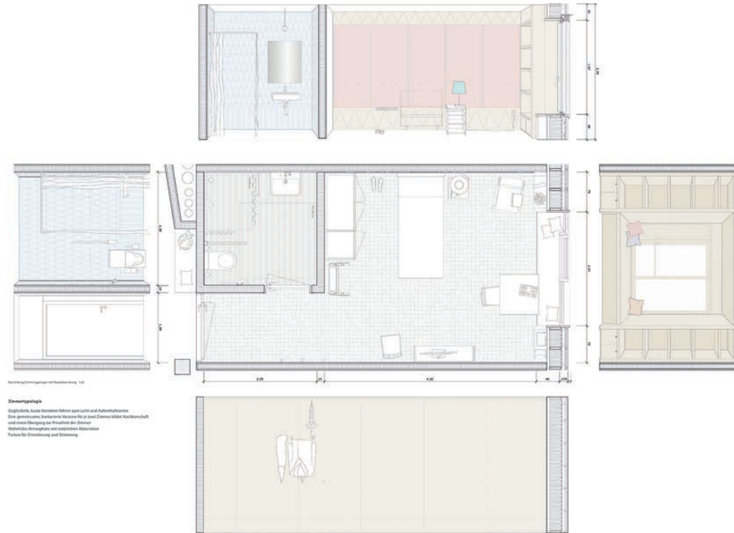
Pflegezimmer 1:100
