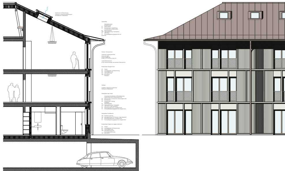
Fassadenschnitt 1:200
