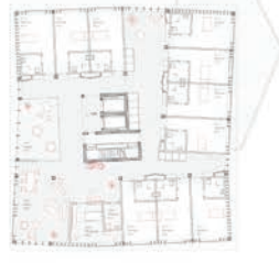
1. Obergeschoss 1:500
