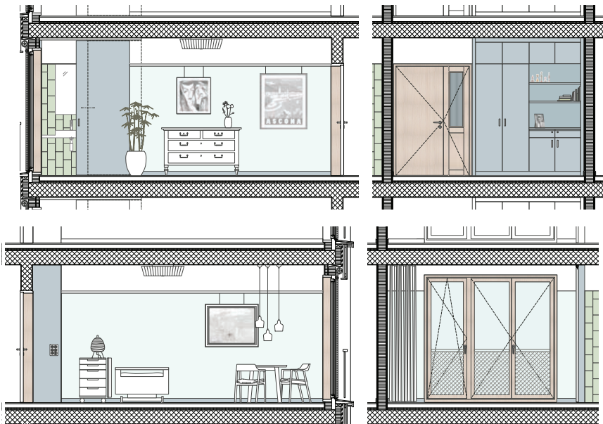
Pflegezimmer Langzeitpflege 1:100
