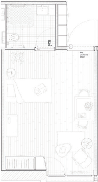
Pflegezimmer 1:100
