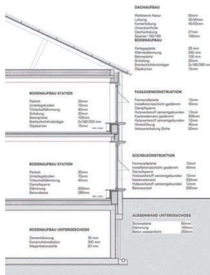
Fassadenschnitt 1:200
