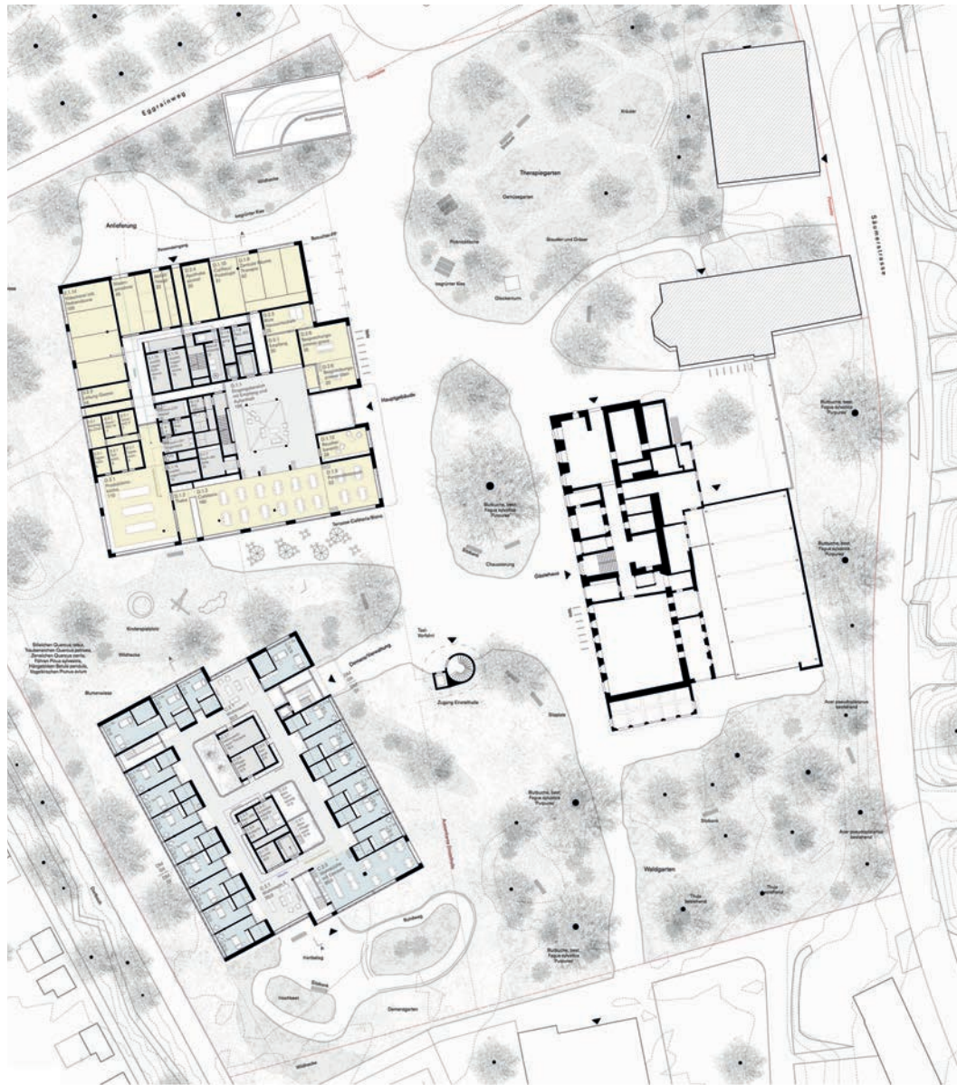
Erdgeschoss 1:1000
