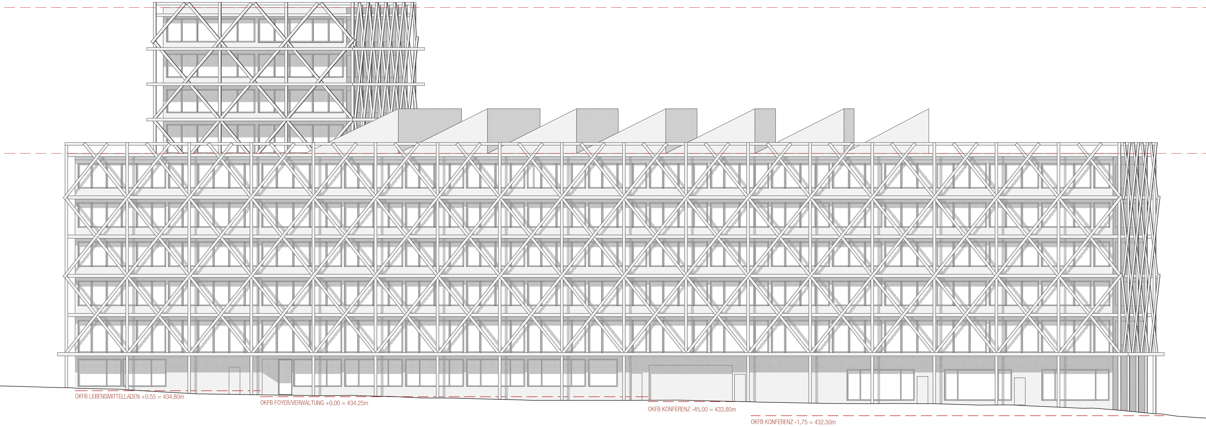
Fassade Seetalstrasse - 1/200
