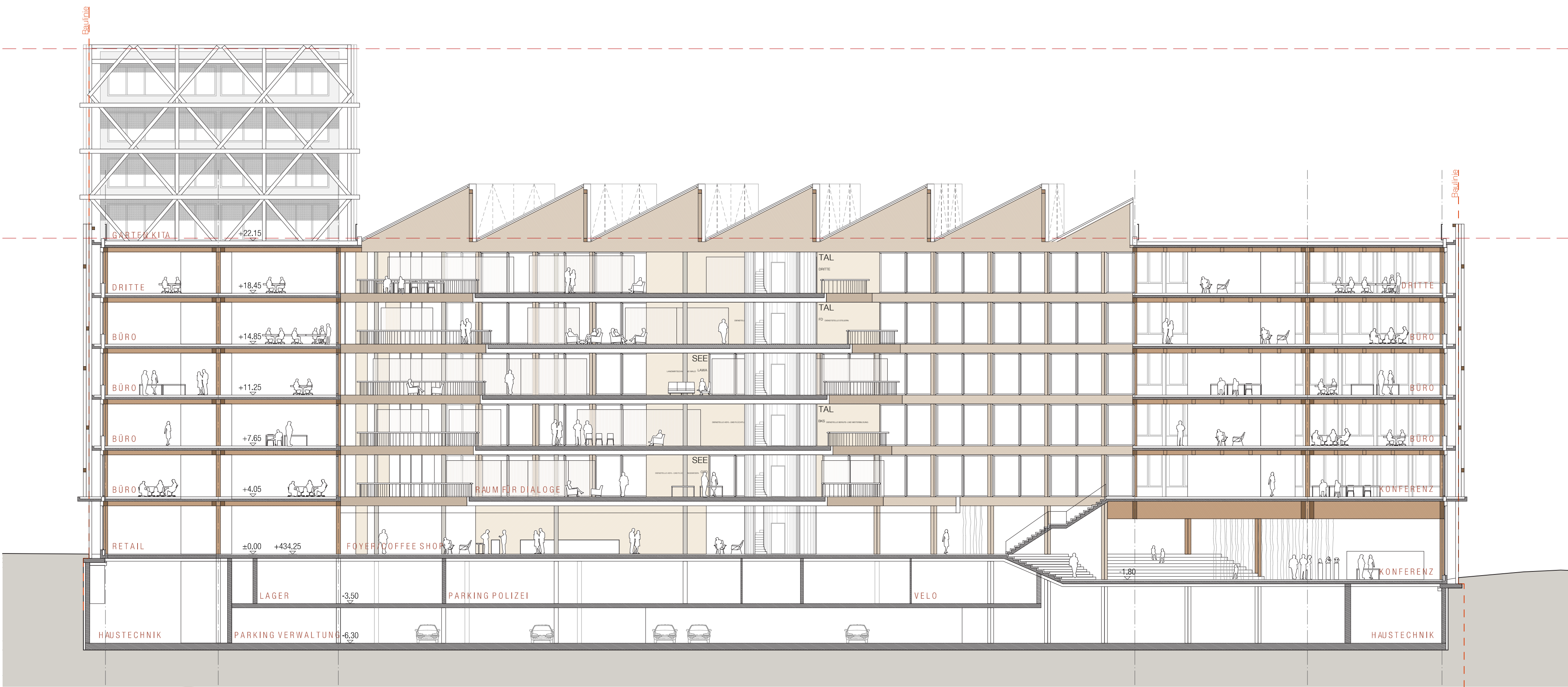
Schnitt A-A - 1/200
