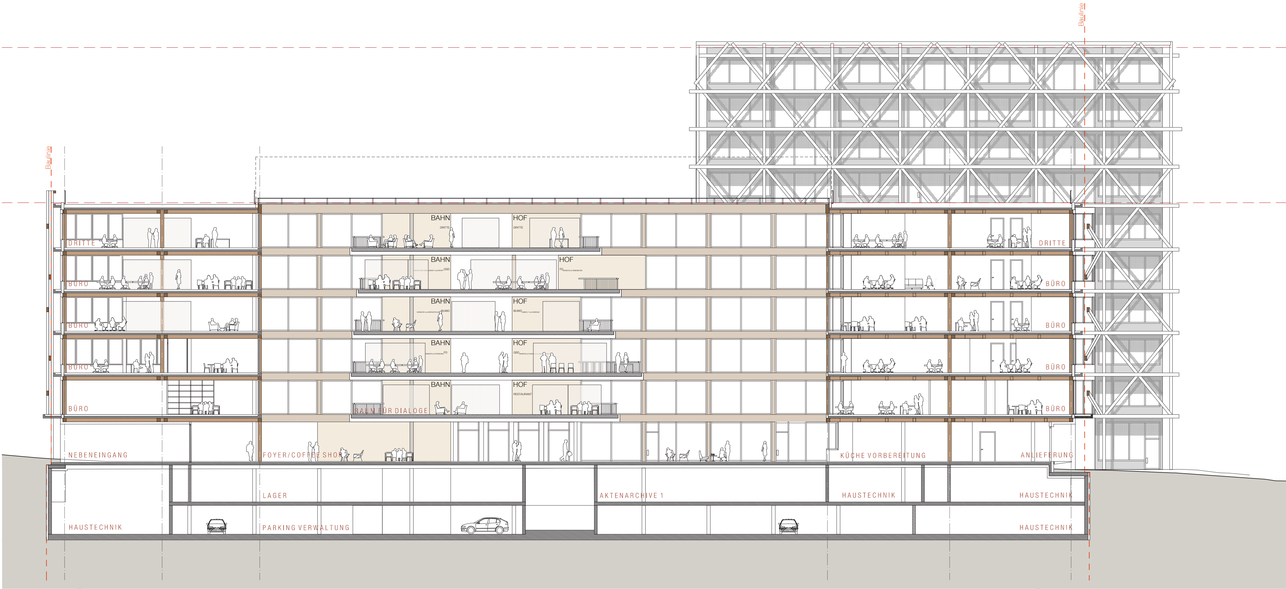
Schnitt B-B - 1/200
