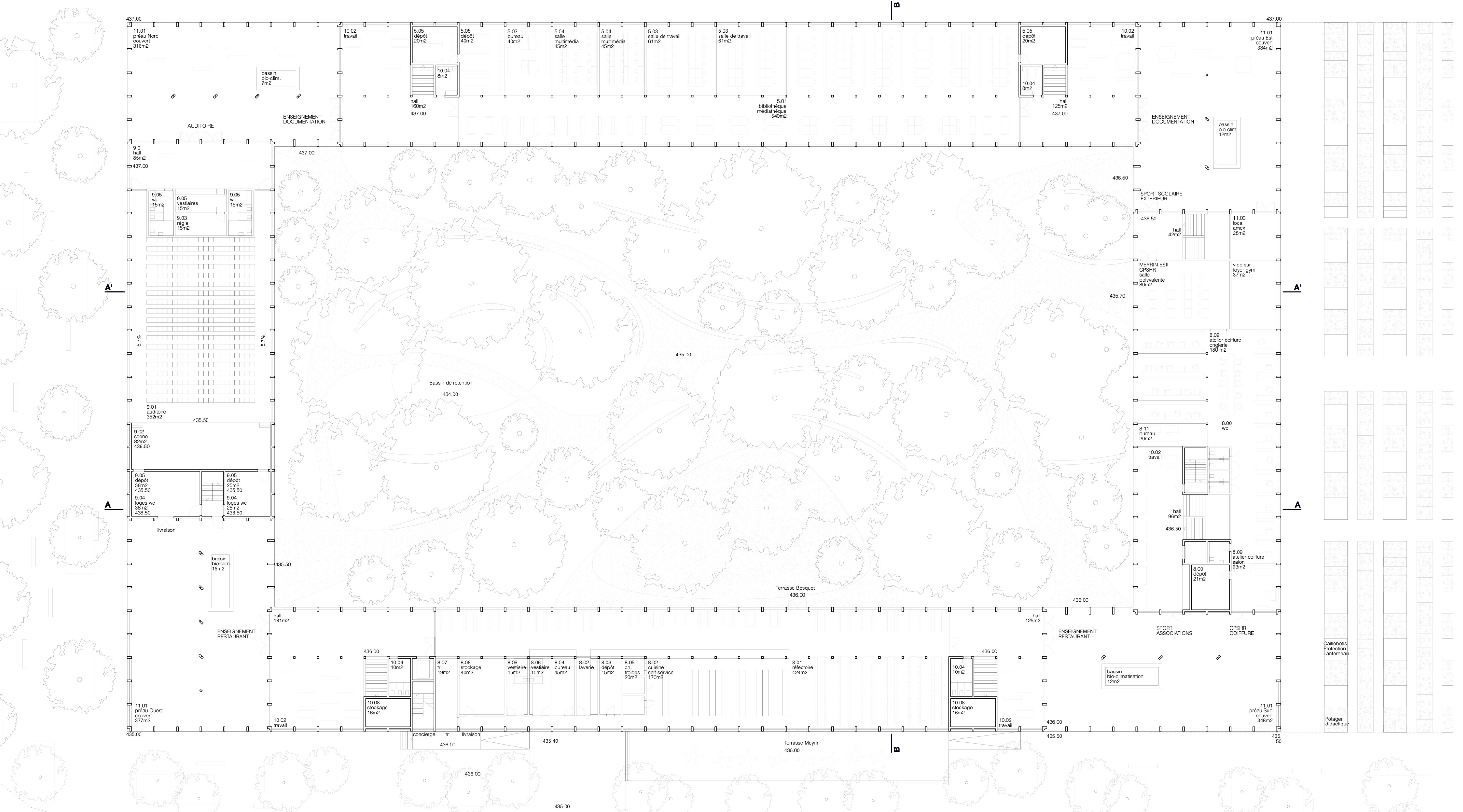
PLAN DU REZ-DE-CHAUSSEE 1:200
