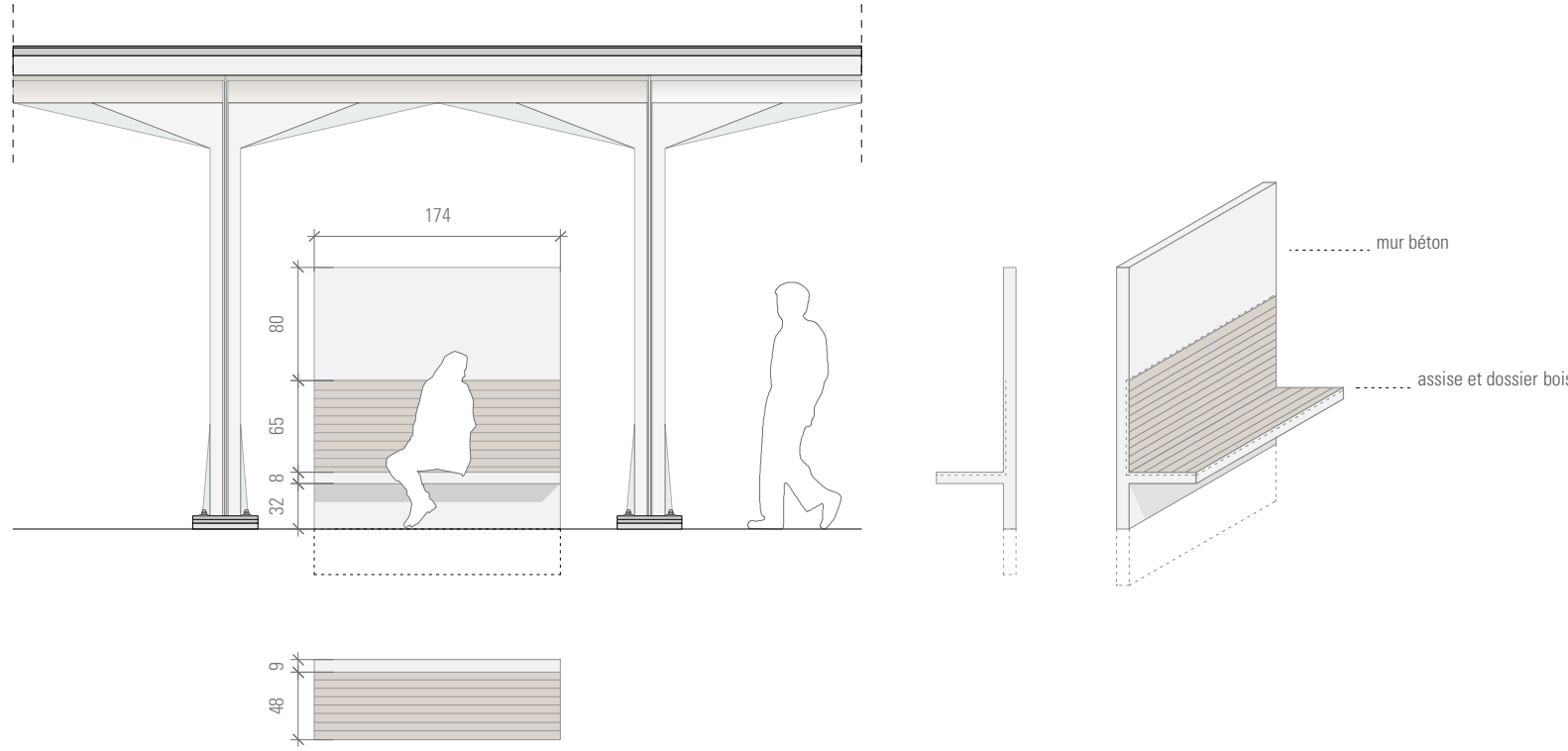
BANC 1:50
