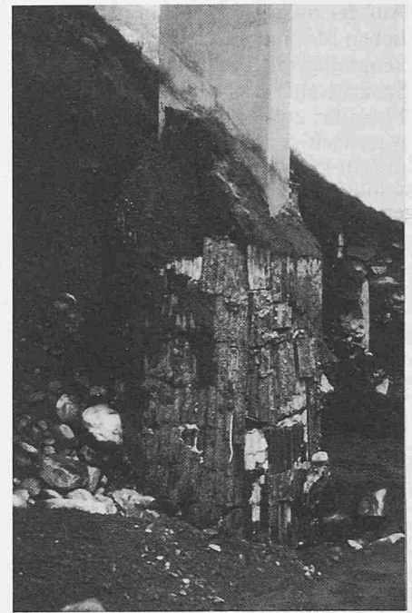
Bild 5. Freigelegtes Schachtfundament
