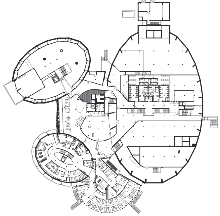
Pianta piano intermedio. Fonte Suisse Projets – Garzoni SA
