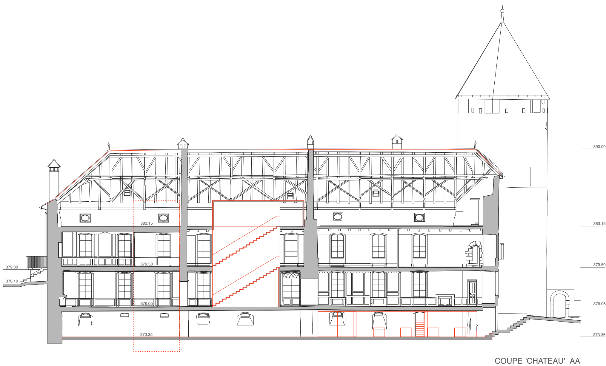
COUPE 'CHATEAU' AA
